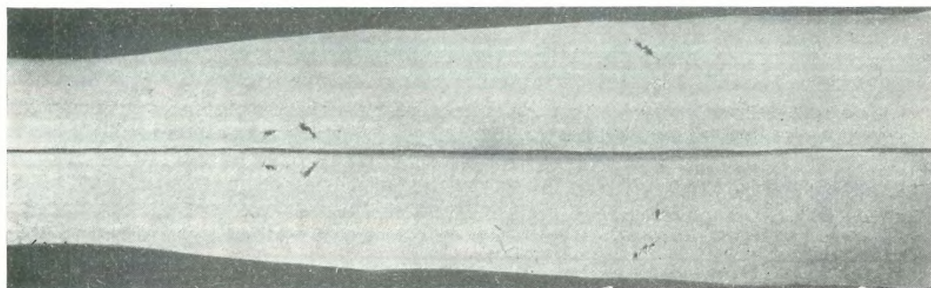
д — незаварившиеся флокены в закаленном изломе
