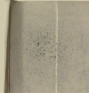
Шкала № 1 Центральная пористость
