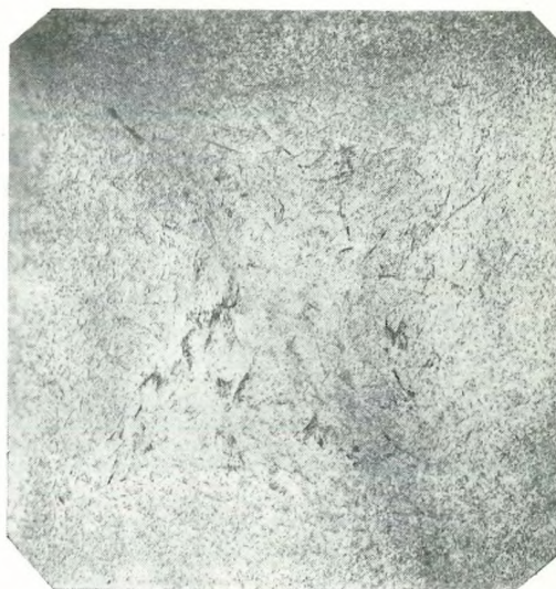
б — церия
