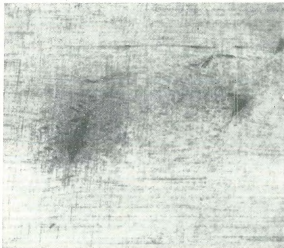
г — незаварившиеся флокены в продольном макротемплете
