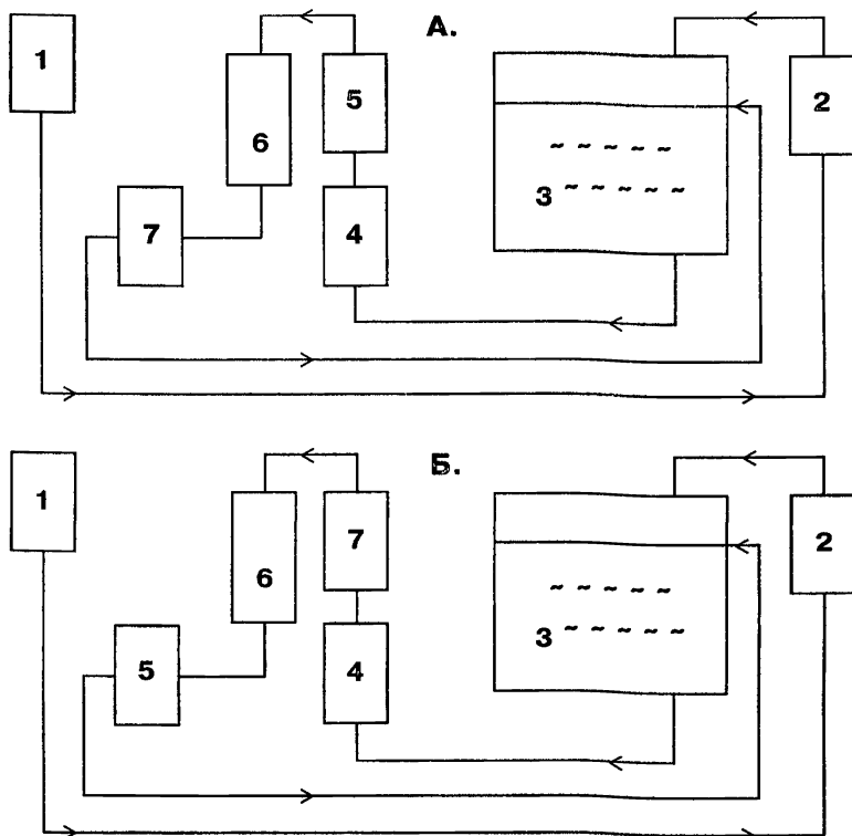
Рис. 2 Принципиальные схемы подключения УФ-установки в бассейнах с системой оборотного водоснабжения
