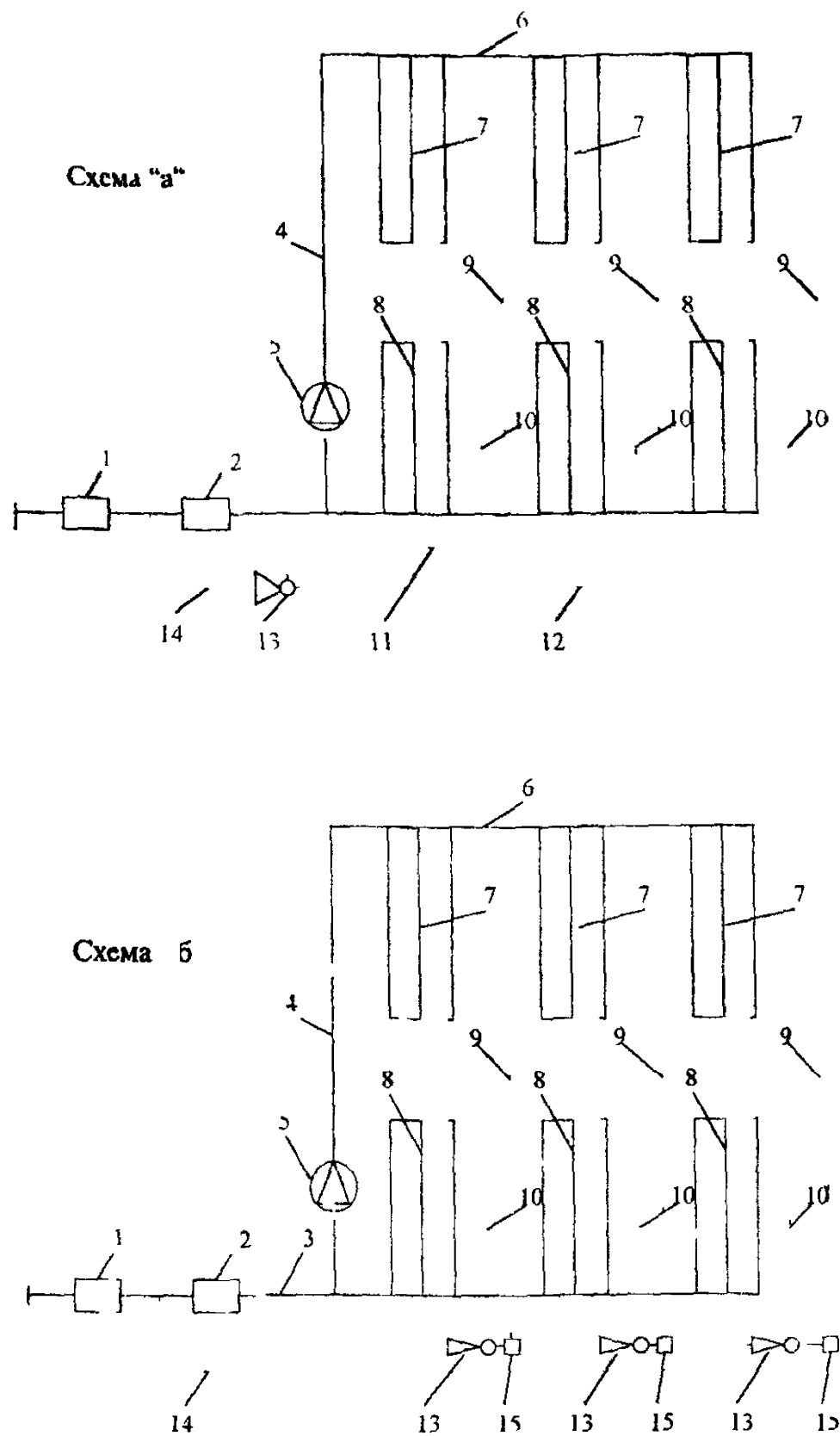
Рис 4 1 Принципиальная схема двухзонной системы горячего водоснабжения с элеваторным побуждением циркуляции в нижней зоне Схемы а с общим элеватором б с элеватором в каждой секции 1 2 водонагреватель первой и второй ступени 3 подающий трубопровод нижней зоны 4 главный стояк верхней зоны 5 повысительно циркуляционный насос верхней зоны 7 8 водоразборные стояки верхней и нижней зон 9 10 циркуляционные стояки верхней и нижней зон 11 12 циркуляционные сборные трубопроводы нижней и верхней зон 13 элеватор 14 общий циркуляционный трубопровод 15 грязевик
