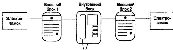
Рисунок 11 - Схема домофона из двух камер и одного монитора
