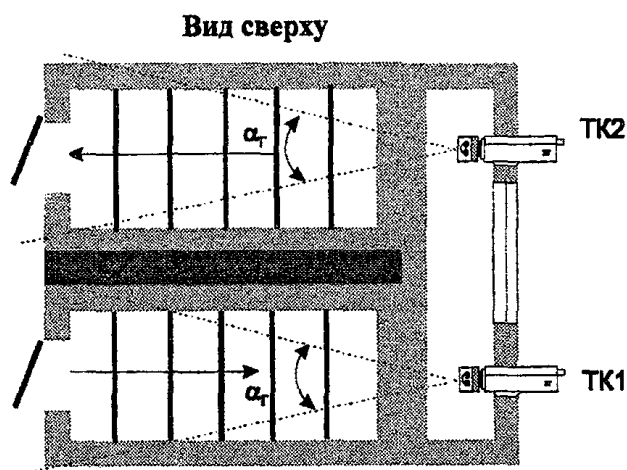
Рисунок 6 – Схемы охраны лестничных пролетов
