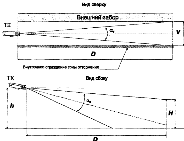
Рисунок 7 - Схемы охраны периметра
