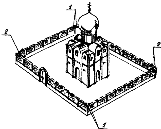
Рис. 10 - Вариант блокировки периметра внешнего ограждения церкви 1 - излучатели извещателей "Рубеж-3М"; 2 - приемники извещателей "Рубеж-3М".
