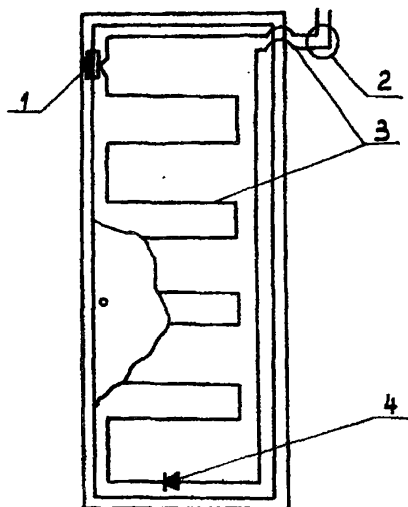
Рис. 11 - Вариант блокировки двери проводом на "пробой" 1 - извещатель СМК-1 (И0102-4); 2 - коробка соединительная К-14; 3 - провод НВМ; 4 - диод.
