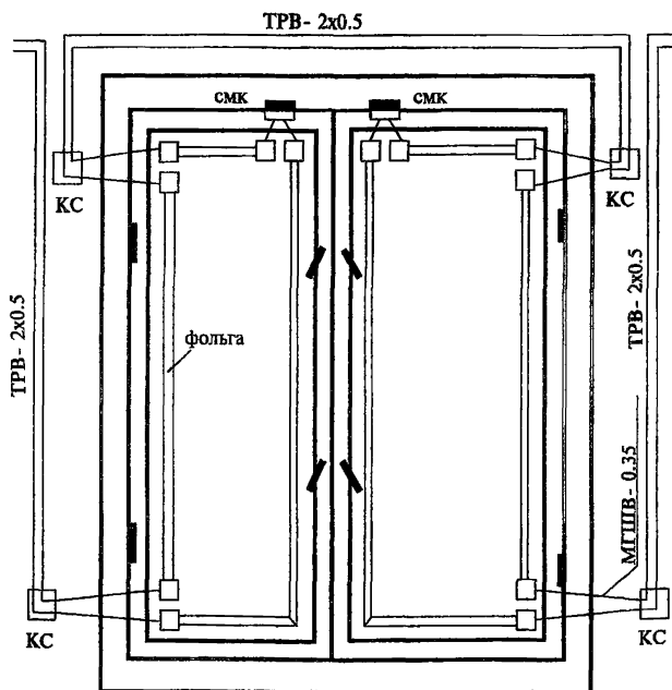
Рисунок 1 - Блокировка окна извещателями омическими типа «Фольга», «Провод» и магнитоконтактными типа СМК
