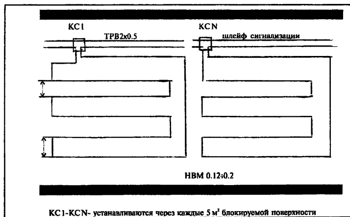
Рисунок 8 - Блокировка стен извещателем омическим типа "Провод"
