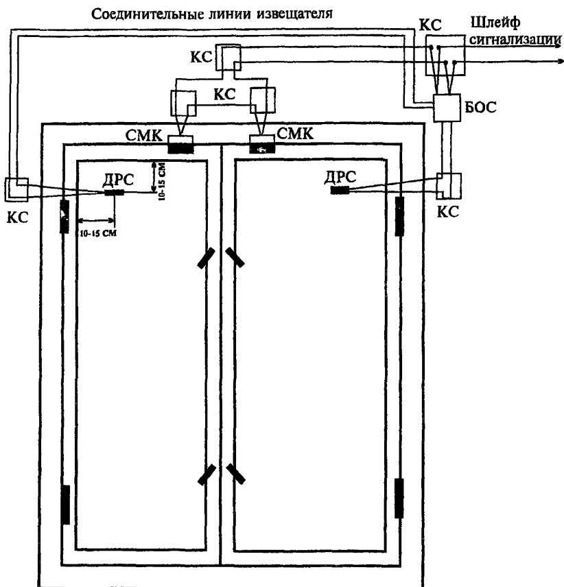
БОС-Блок обработки сигнала извещателя "Окно-4" ДРС-Датчик разрушения стекла
