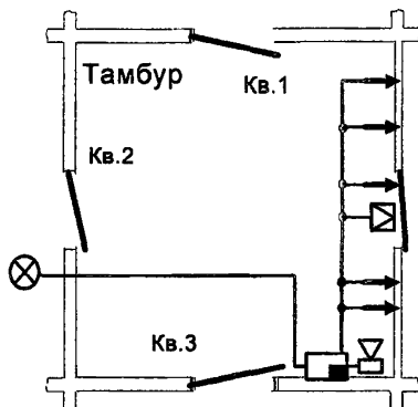
Рисунок 11 - Солидарная охрана двери квартирного тамбура
