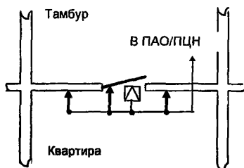
Рисунок 15 - Автономная (централизованная) охрана входной двери квартиры
