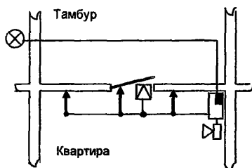
Рисунок 14 - Солидарная охрана входной двери квартиры
