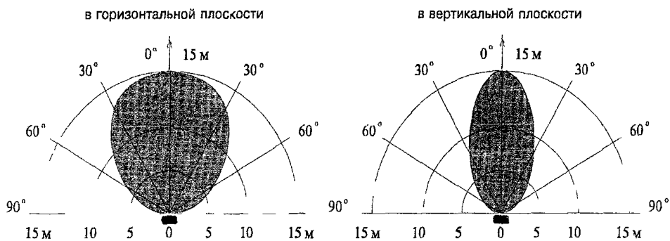
Рисунок 3 52 - Извещатель "Тюльпан-3"
