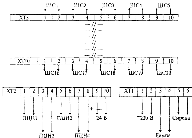
Рисунок 4.25 - "Пульсар"
