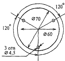
Рисунок 3 6 - "Эхо-2"
