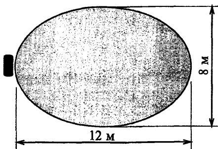
Рисунок 3.51 - Извещатель "Волна-5"
