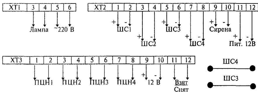
Рисунок 4 17 - "Сигнал-ВК-4"
