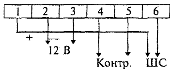
Рисунок 3.30 - "Тюльпан-3"
