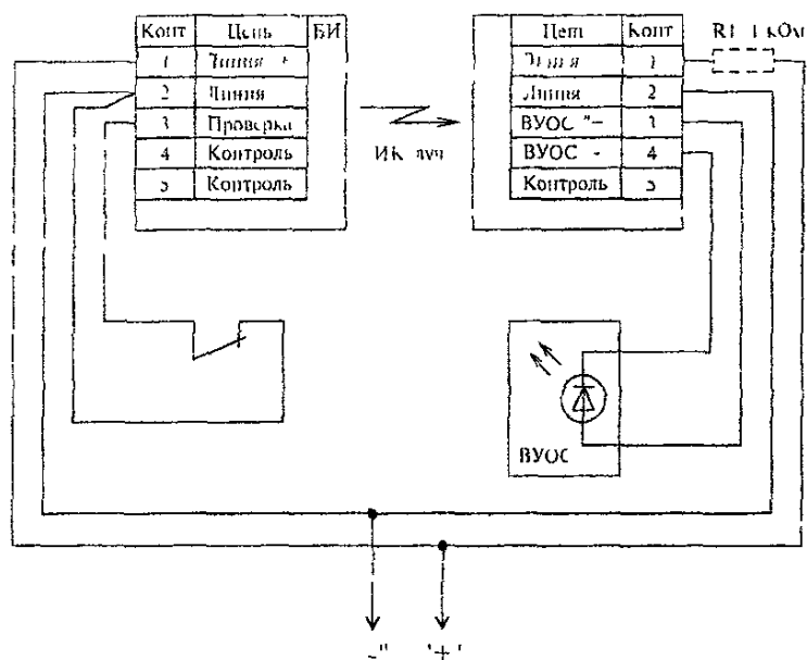
Рисунок 7.7 - Извещатель ИП 212-7 “ИДПЛ”
