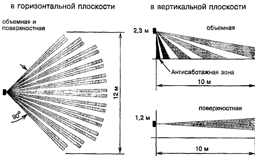
Рисунок 3.48 - Извещатель "Фотон-СК"
