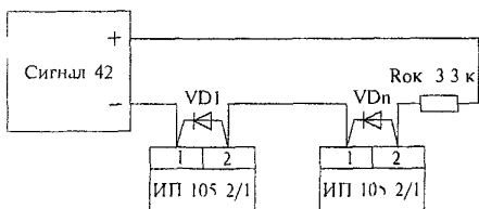
Рисунок 7 5 - Извещатель ИП 105-2/1
