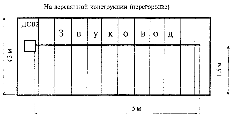
Рисунок 6.25 - Блокировка стен, потолка и пола на пролом извещателем поверхностным "Грань-2"
