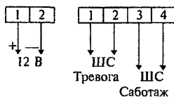
Рисунок 3.28 - "Фотон-СК"
