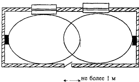
Рисунок 6 30 - Блокировка помещения несколькими радиоволновыми, ультразвуковыми и комбинированными извещателями
