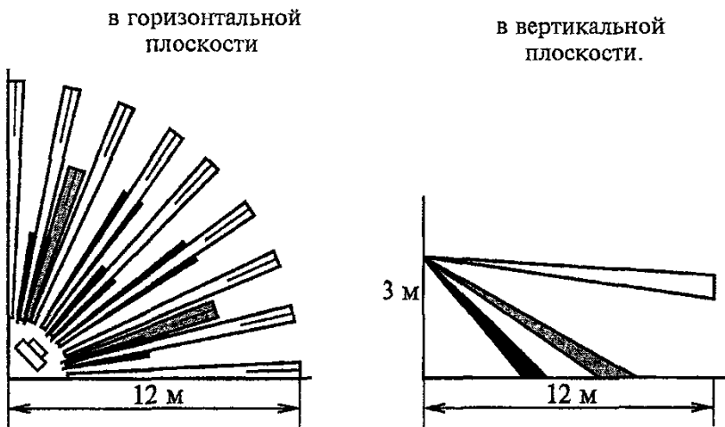
Рисунок 3.42 - Извещатель “Фотон-4”
