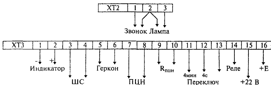
Рисунок 4.15 - "Сигнал-45"
