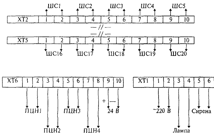
Рисунок 4.23 - "Рубин-6"
