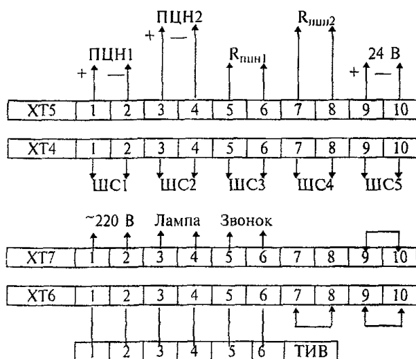
Рисунок 4.19 - "Квинта"
