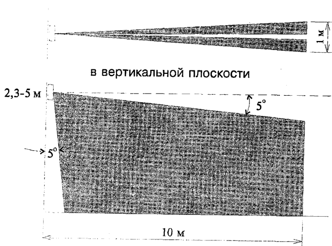
Рисунок 3.43 - Извещатель "Фотон-5"
