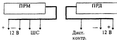
Рисунок 3.33 - “Радий-2”, “Радий-2/1”, “Радий-2/2”
