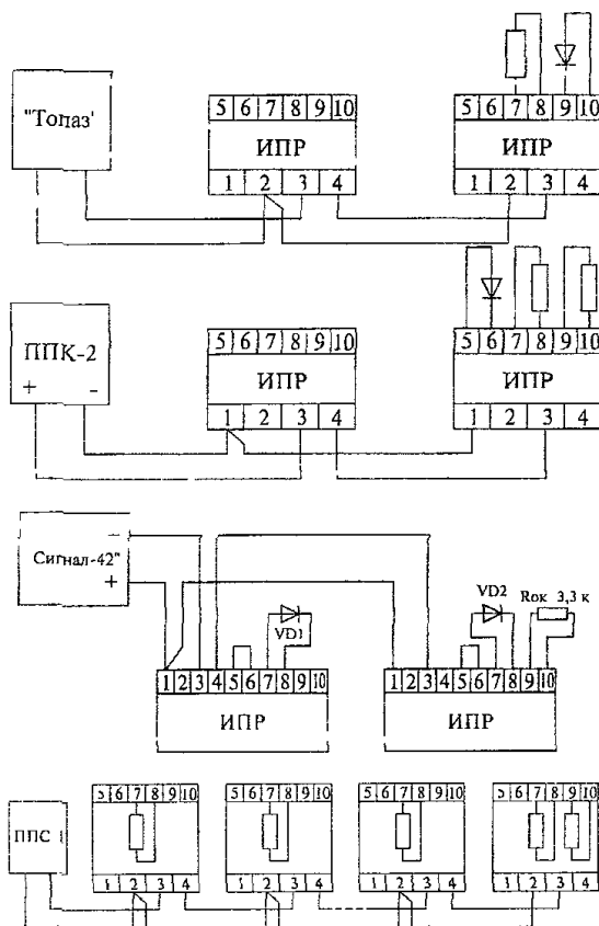
Рисунок 7.9 - Извещатель ИПР
