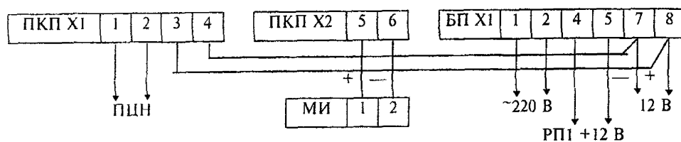
Рисунок 4.21 - "Интервал"
