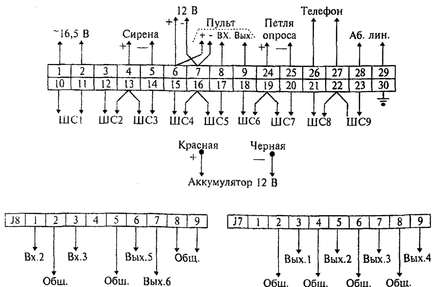
Рисунок 4.29 - "Vista-501"
