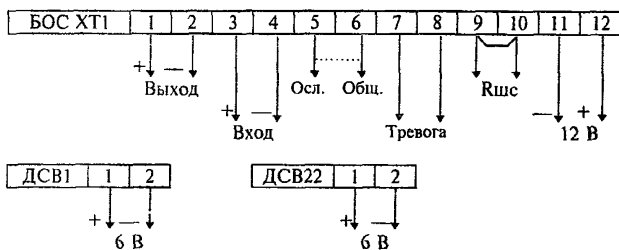
Рисунок 3.15 - "Грань-2"
