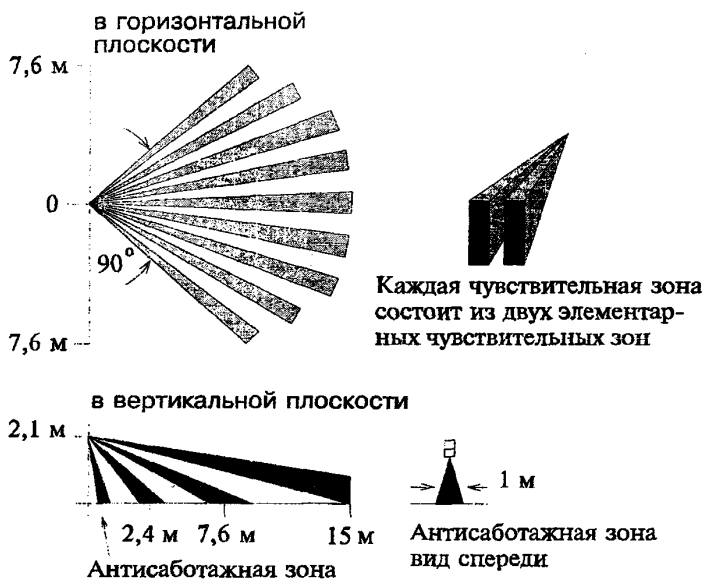
Рисунок 3.47 - Извещатель "9981"
