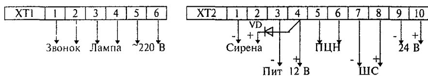
Рисунок 4.16 - "Сигнал-ВК", "Сигнал-ВК-Р"
