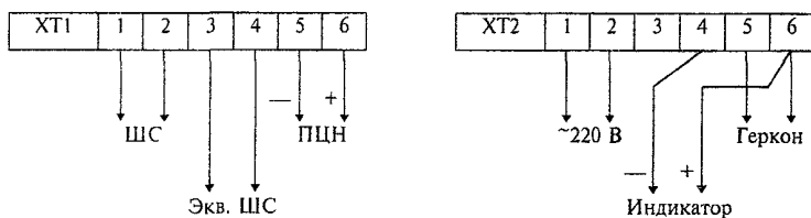
Рисунок 4.13 - "Сигнал-41М"
