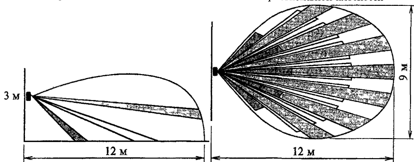
Рисунок 3.57 - Извещатель “Сокол-1”
