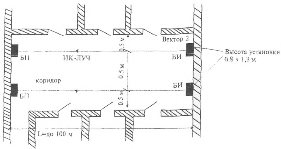
Рисунок 6.37 - Блокировка коридора извещателями линейными активными оптико-электронными
