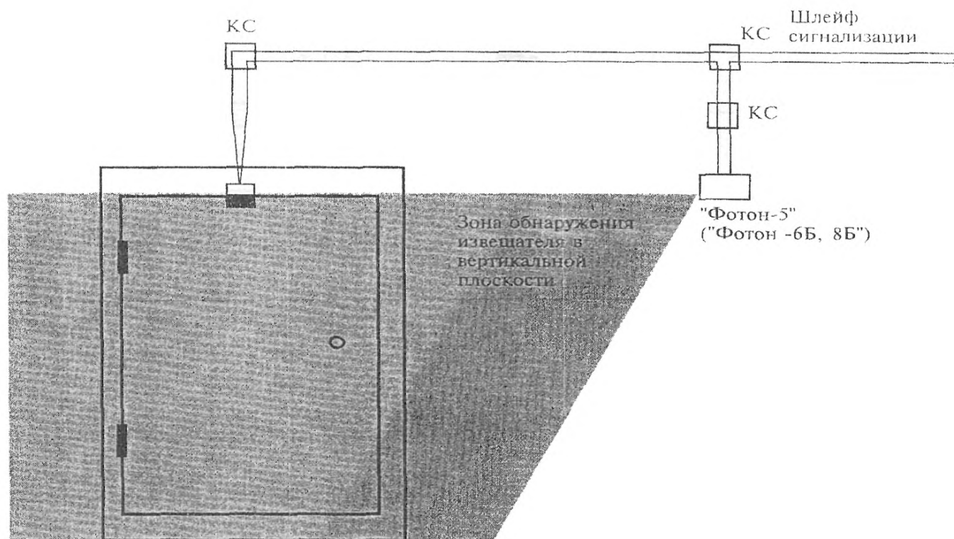
Рисунок 6.13 - Блокировка двери на открывание и проникновение извещателями магнитоконтактными и пассивными оптико-электронными с зоной обнаружения типа "занавес"
