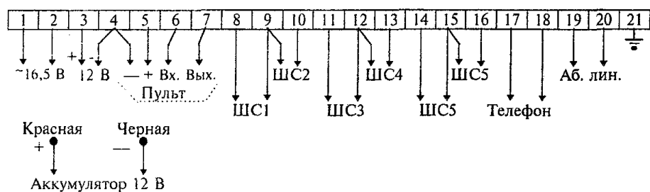
Рисунок 4.26 - "Vista-101"
