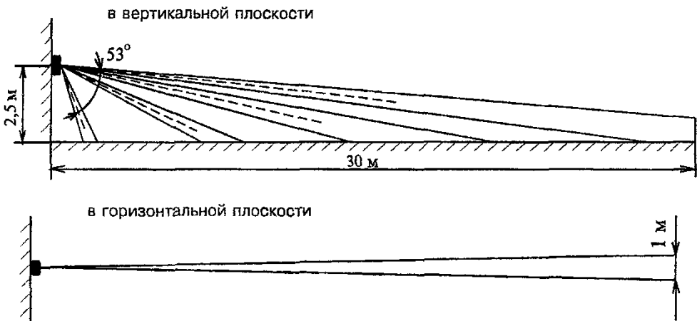
Рисунок 3.41 - Извещатель “Фотон-2”
