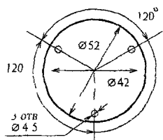
Рисунок 3 7 - "Эхо-3"
