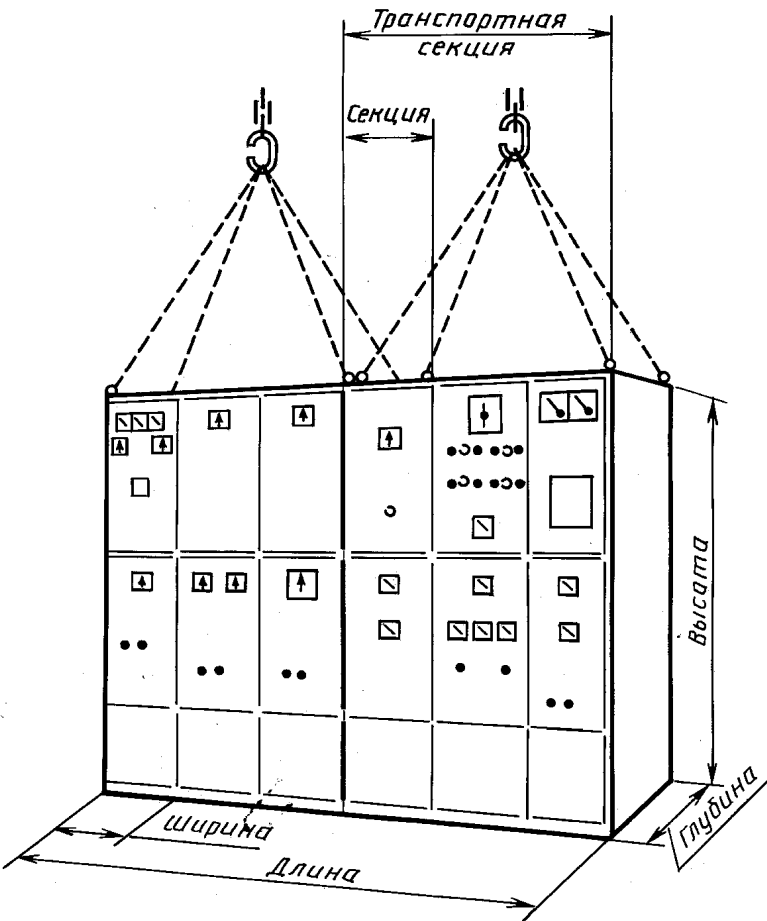
НКУ заводского изготовления многоящичного типа Черт. С.4
