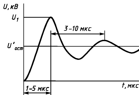
Рисунок Д.3 — Форма грозовых импульсов, характерная для точек присоединения, проходящих через выводы силового трансформатора, рассматриваемая обмотка которого имеет связь с ВЛ (точки присоединения z , z' , u на рисунке Д.1)
