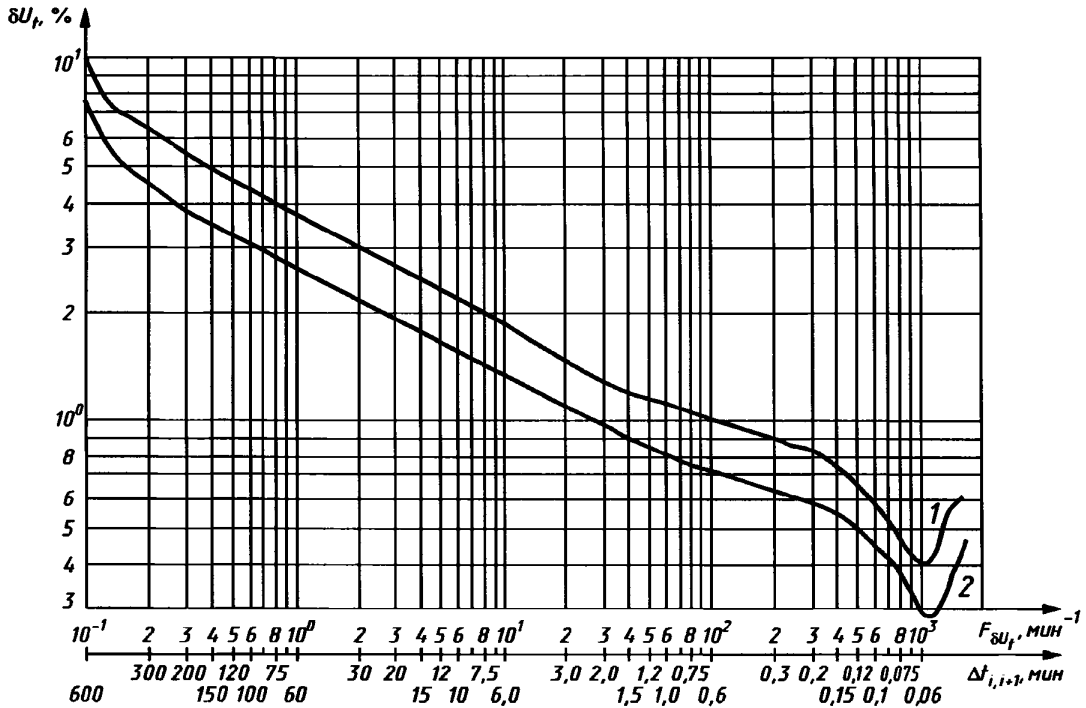
Рисунок 1 — Предельно допустимые размахи изменений напряжения в зависимости от частоты повторения изменений напряжения за минуту для колебаний напряжения, имеющих форму меандра
