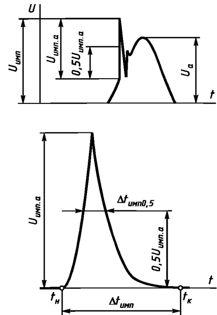
Рисунок Б.3 — Параметры импульсного напряжения
