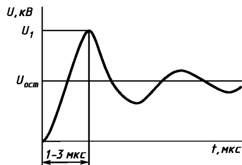
Рисунок Д.2 — Форма грозовых импульсов, характерная для точек присоединения a , b , z , д на рисунке Д.1.
