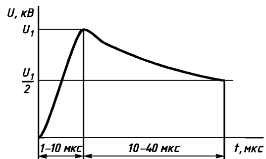
Рисунок Д.4 — Форма грозовых импульсов, характерная для точек присоединения b , e , ж на рисунке Д.1.
