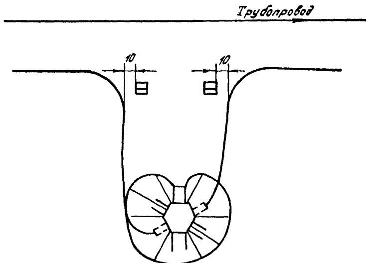
Рис.2I. Установка дополнительных столбиков у НУПа
