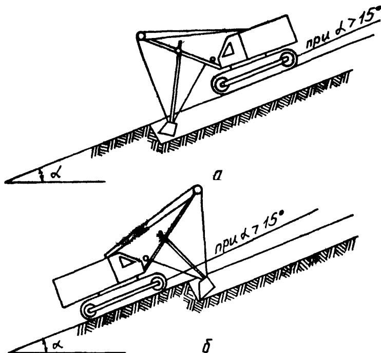
Рис.8. Схема работы на уклоне одноковшового экскаватора: а – с прямой лопатой; б – с обратной лопатой
