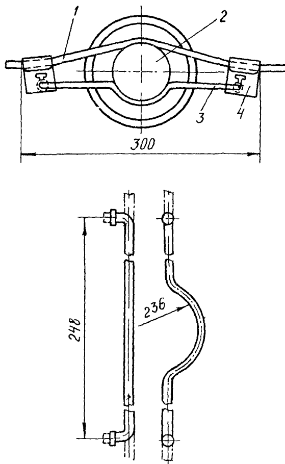
Рис.33. Антивибрационный крововый зажим ЗАК-Ю-І: І - провод; 2 - изолятор; 3 - скоба; 4 - захватывающая скоба
