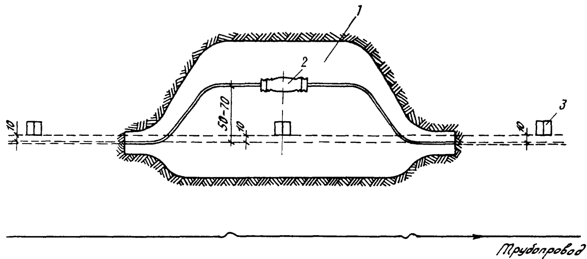
Рис.15. Установка замерного столбика у муфты на однокабельной линии связи: 1 - котлован; 2 - муфта; 3 - замерный столбик
