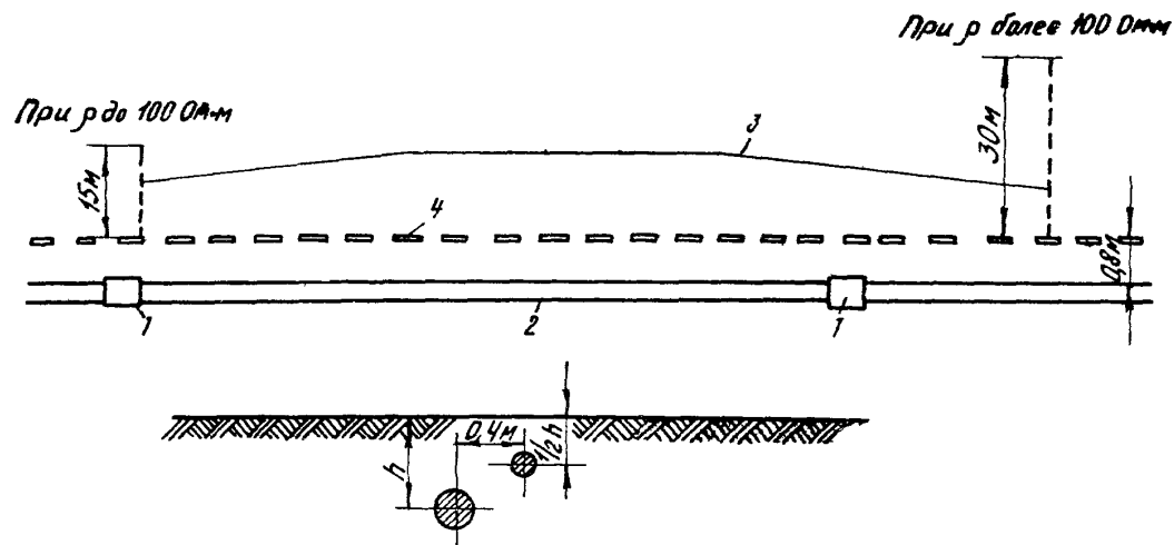
Рис.24. Схема прокладки одного защитного провода (троса): 1 - муфта; 2 - кабель; 3 - лучевой заземлитель; 4 - защитный провод
