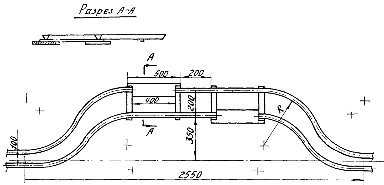
Рис. 23. Рама для закрепления выкладки кабеля
