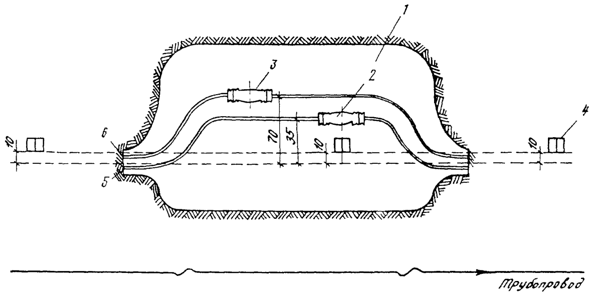
Рис.16. Установка замерного столбика у муфт на двухкабельной линии связи: 1 - котлован; 2 - муфта № 1; 3 - муфта № 2; 4 - замерный столбик; 5 - кабель № 1; 6 - кабель № 2
