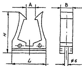
Рис. 10. Схема пластмассовых клищ типа Л 75УЗ-Л178УЗ для крепления пластмассовых труб для электропроводок
