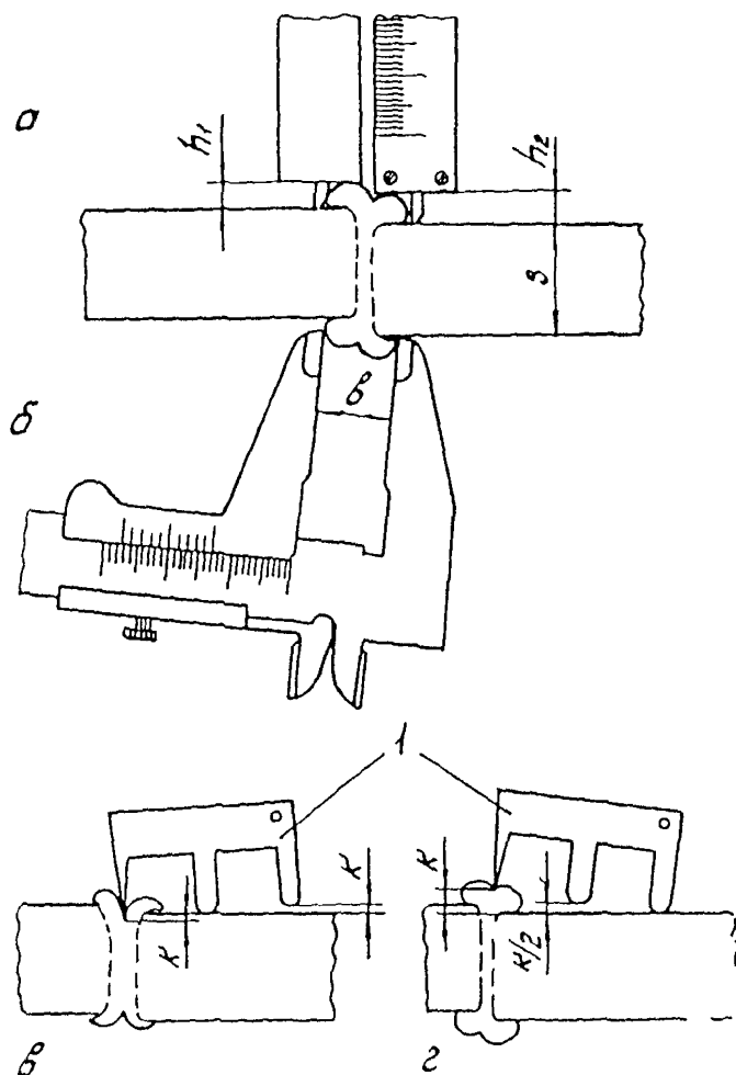
Рис.15. Схема измерения параметров стыкового соединения: а - высота валиков грата h_1, h_2 ; б - ширина грата \delta ; в, г - величина усиления К (случай "в" - брак); 1 - приспособление для определения К с помощью щупа
