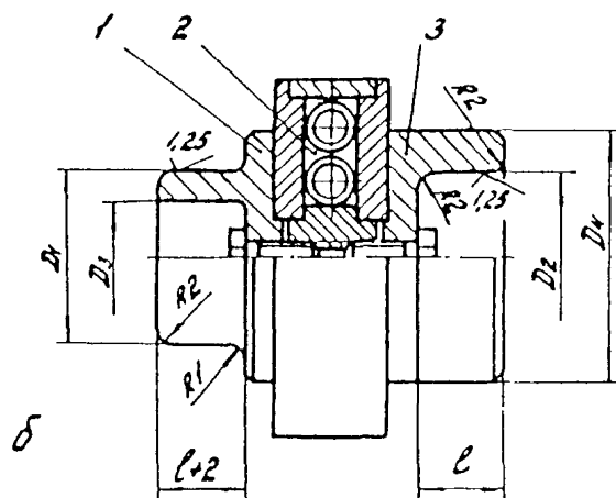
Рис.10. Схема нагревательного инструмента для раструбно-стыковой сварки;
