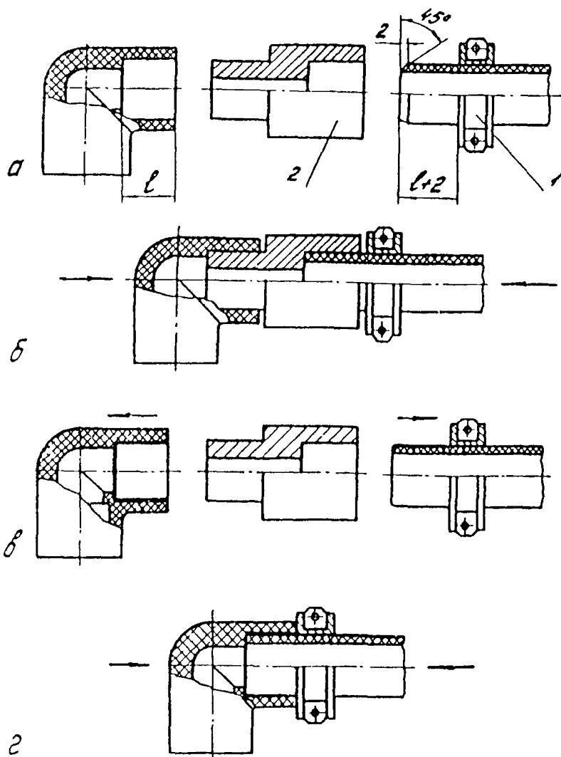
Рис. 9. Последовательность процесса контактной сварки впастроб труб и соединительных деталей из ПВД: а - центровка, закрепление в зажимах сварочного устройства концов свариваемых труб и деталей и установка ограничительного хомута 1; б - установка дорна нагретого инструмента 2 в раструбе и гладкого конца трубы в гильзе; в - нагрев (оплавление) свариваемых концов, одновременно снятие их с дорна и гильзы; г - соединение концов с выдержкой до затвердевания сплавленного материала
