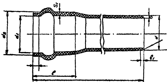
Рис. 2. Напорная раструбная труба из ПЕХ (размеры см. табл.3)
