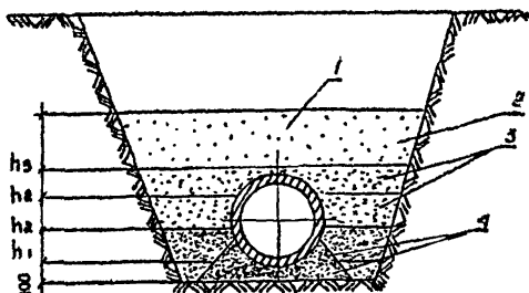
Рис. 6. Схема уплотнения грунта при засышке траншеи с канализационным трубопроводом из ПВХ:
