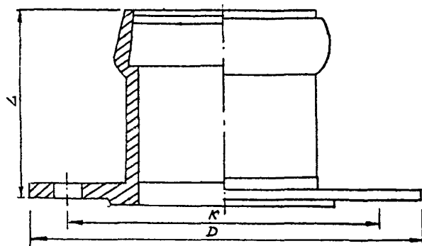
Фланец - раструб Е - К S
