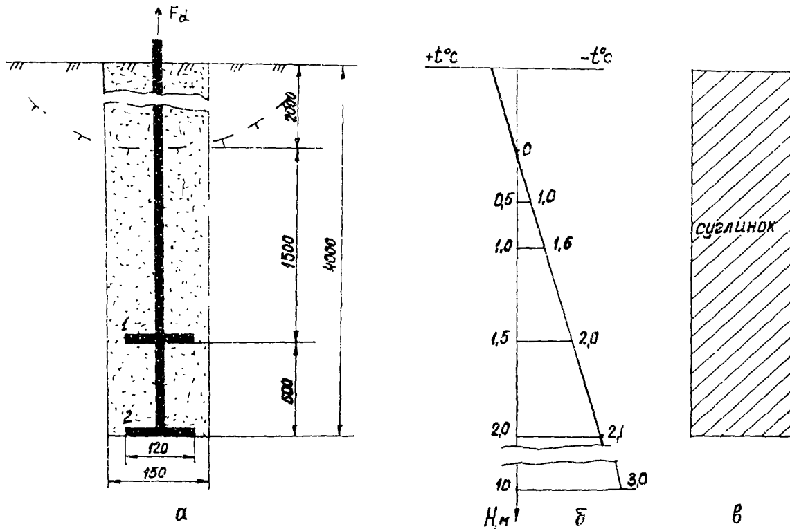
Схема к расчету двухстадийного анкера: а - схема анкера; б - расчетная температура грунта; в - геологический разрез участка
