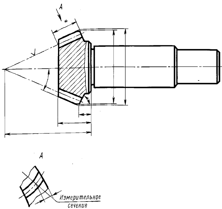
Пример указания параметров зубчатого венца на чертеже конического зубчатого колеса с круговыми зубьями со стандартным исходным контуром
