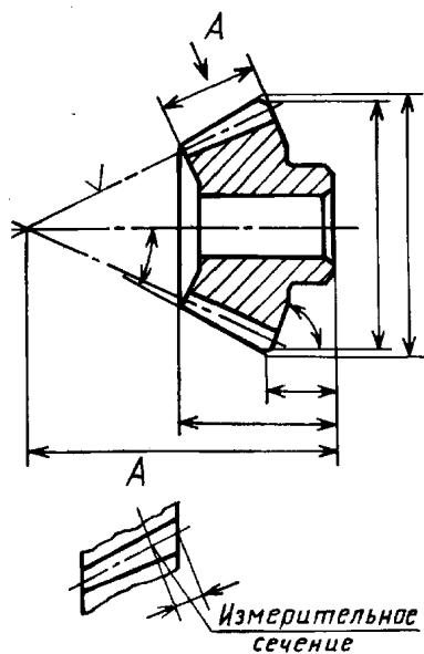
Пример указания параметров зубчатого венца на чертеже конического зубчатого колеса с тангенциальными зубьями со стандартным исходным контуром
