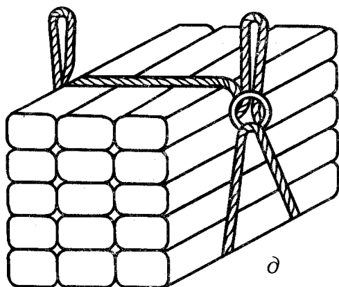
a — скрепление при помощи строп УСК; б — скрепление при помощи строп СПО-4; в, д — гибкие пакетирующие стропы; z — металлическая стяжка; e — кассета
