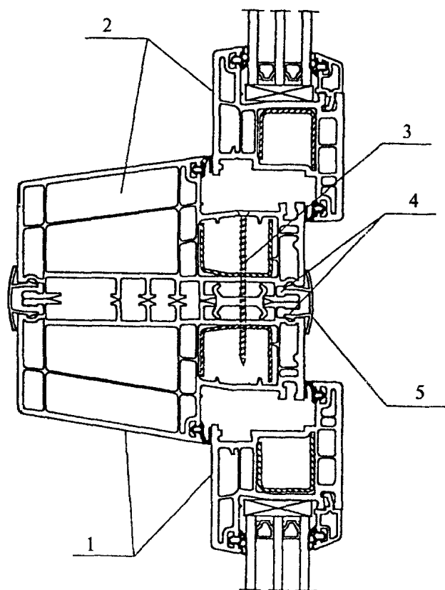
1 — оконный блок; 2 — дверной балконный блок; 3 — стяжной шуруп; 4 — силиконовый герметик; 5 — нагельник
