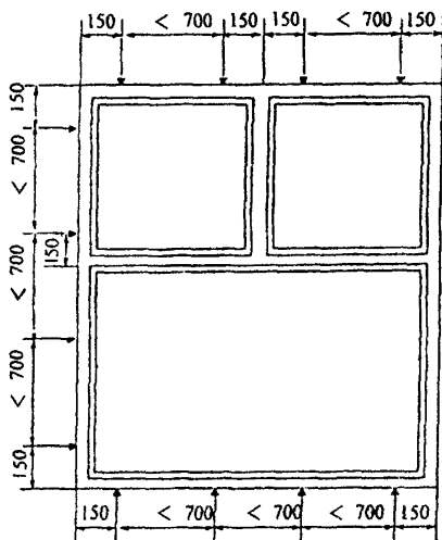
Рисунок Г.3 — Расположение крепежных деталей
