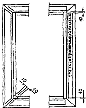
Рисунок 6 — Примеры установки усилительных вкладышей
