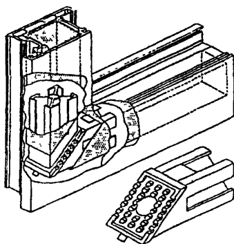
Рисунок 7 — Вкладыш для усиления угловых соединений
