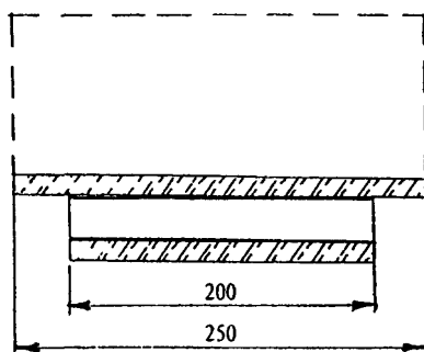
Рисунок 8 — Испытание герметика первого герметизирующего слоя
