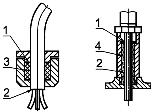
1 — место ввода кабеля; 2 — место разделки жил кабеля; 3 — уплотнительное кольцо; 4 — герметизирующий компаунд
