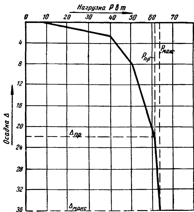
График зависимости осадки сваи \Delta в мм от нагрузки P в т ( P_{\max} и \Delta_{\max} — соответственно нагрузка и осадка, достигнутые в конце опыта)
