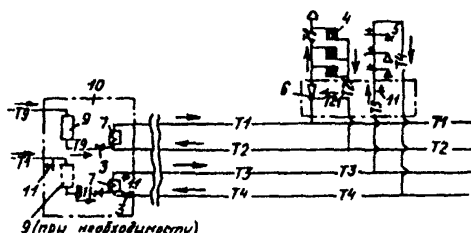
Рис. 3. Схема теплоснабжения с отдельными сетями горячего водоснабжения
