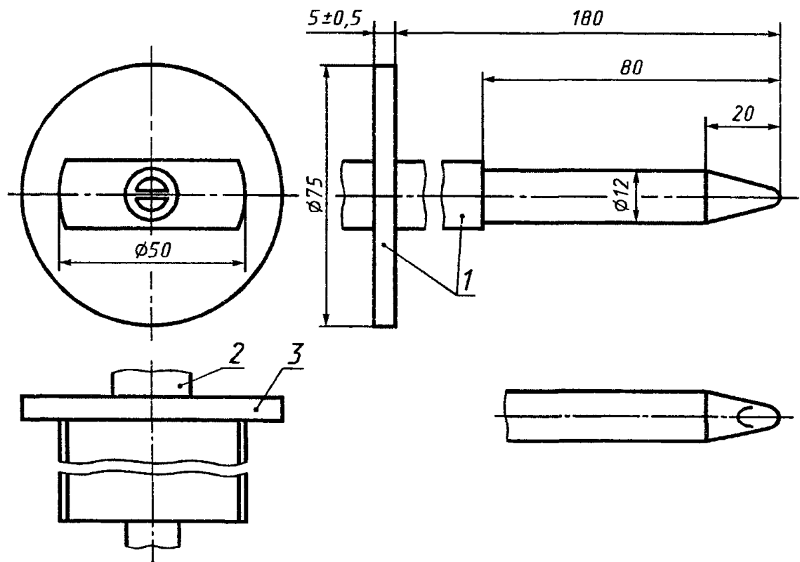
Рисунок Г 1 — Шарнирный испытательный палец
