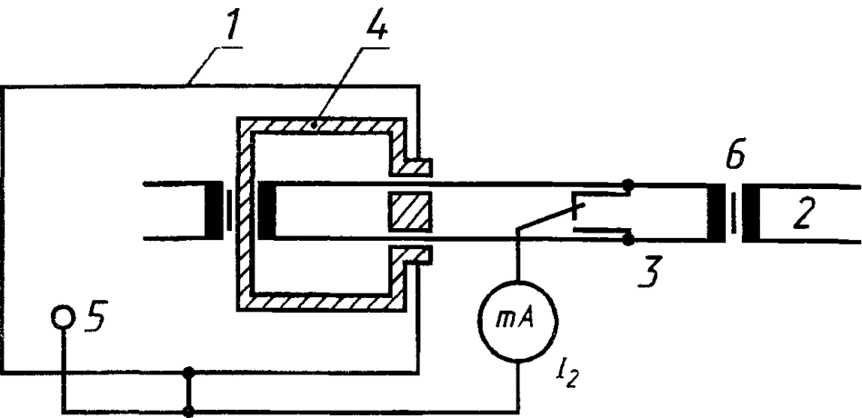
Рисунок Ж 2 — Схема для измерения силы тока утечки аппаратов группы II 2
