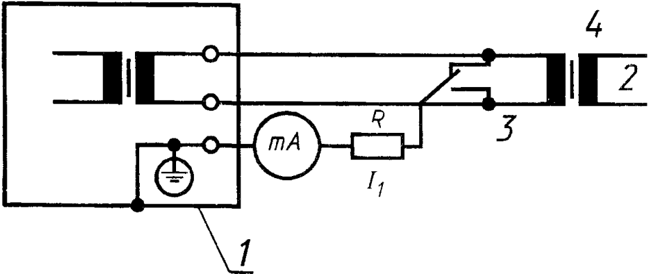
Схема цепи для измерения силы тока утечки
