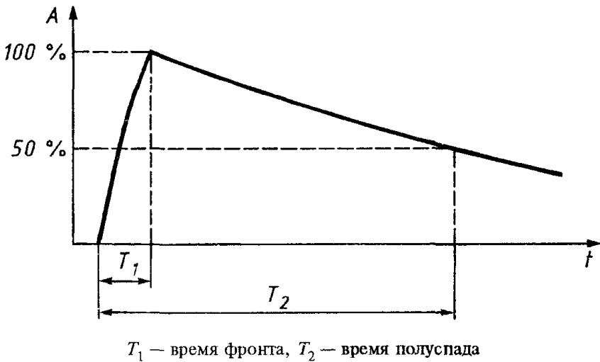
Рисунок Е 2 — Форма грозового импульса и импульса перенапряжения по линии связи
