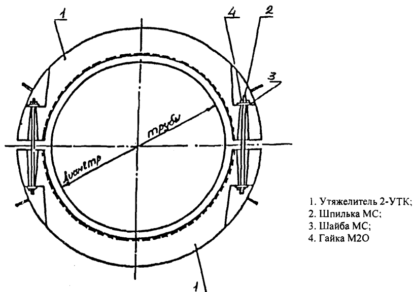
Рис. 1. Железобетонный утяжелитель типа 2 - УТК
