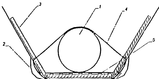
Рис. 8. Железобетонный утяжелитель типа УБГ: 1 - газопровод; 2 - приямок в траншее для установки утяжелителя; 3 - шарнирно-соединенные плиты; 4 - силовой соединительный пояс; 5 - дно траншеи
