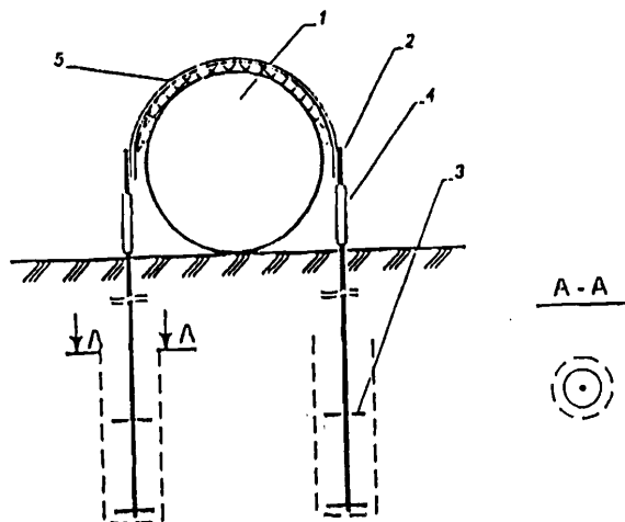
Рис. 12. Дисквое вмораживаемое анкерное устройство ДАУ-02К: 1 - газопровод; 2 - тяга; 3 - диск; 4 - ограничитель усилий; 5 - силовой соединительный пояс
