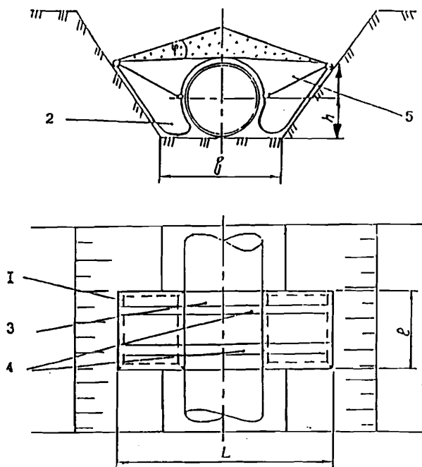
Рис. 3. Схема конструкции полимерно-контейнерного балластирующего устройства:
