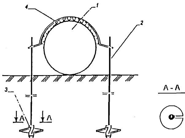
Рис. 10. Винтовое анкерное устройство ВАУ-1: 1 - газопровод; 2 - тяга анкера с наконечником; 3 - винтовая лопасть; 4 - силовой соединительный пояс
