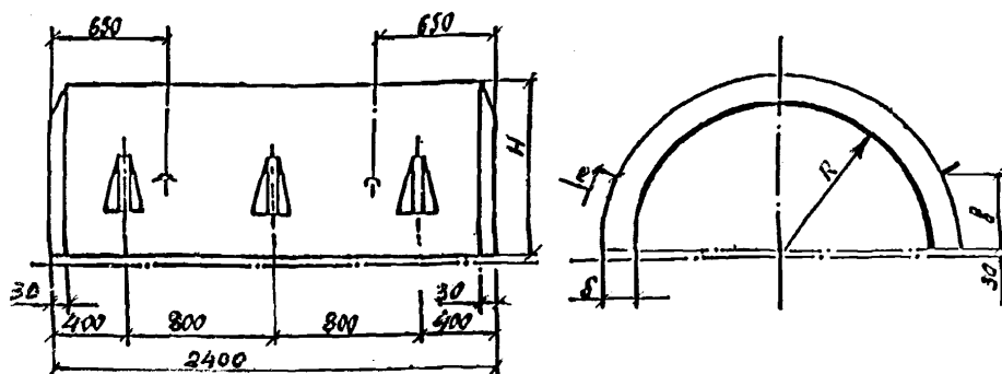
Рис. 1. Железобетонный утяжелитель типа 2 - УТК
