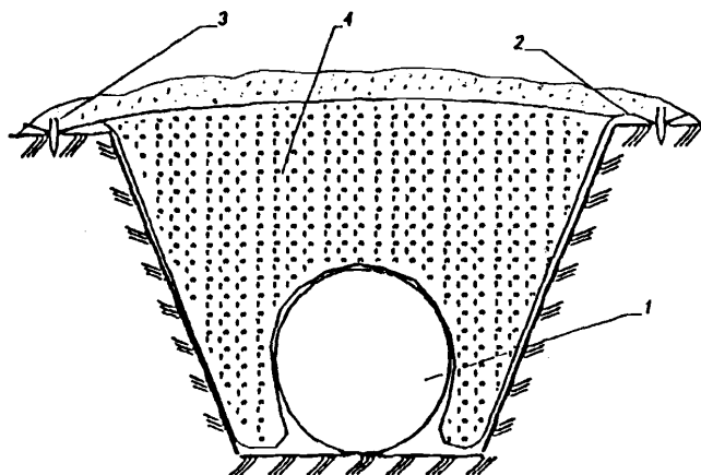
Рис. 14. Способ балластировки газопроводов минеральным грунтом засыпки с использованием полотнищ из HCM (для песчаных грунтов) - схема 1: 1 - газопровод; 2 - полотнище из HCM; 3- металлический штырь; 4 - грунт засыпки
