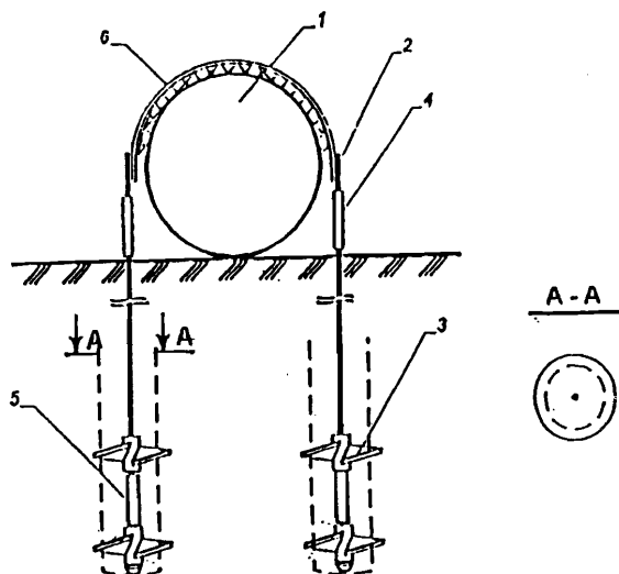
Рис.13. Винтовое вмораживаемое анкерное устройство БАУ-В: 1 - газопровод; 2 - тяга с наконечником; 3 - винтовая лопасть на втулке; 4 - втулка (разделительная); 5 - ограничитель усилий; 6 - силовой соединительный пояс.
