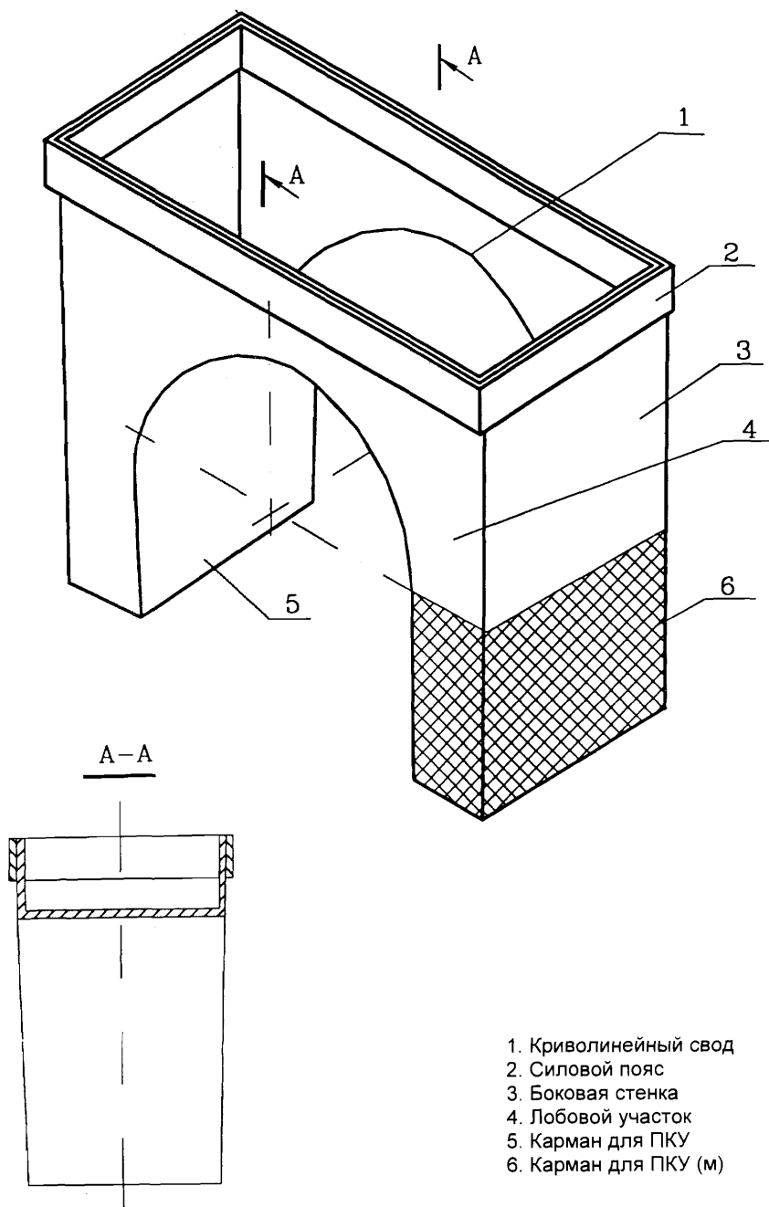
Рис. 18. Полимерконтейнер ПКУ
