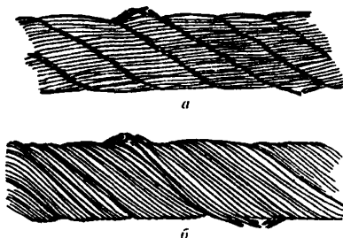
Рис. 2. Сочетание обрывов проволок с их износом:
