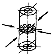
Рис.6. Горизонтальное положение при вертикальном расположении оси свариваемых труб
