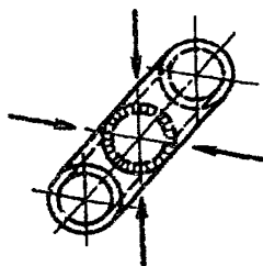
Рис.7. Переменное положение при горизонтальном расположении оси труб, свариваемых без поворота
