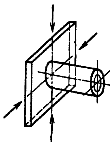
Рис.14. Переменное положение при горизонтальном расположении оси трубы, привариваемой без поворота
