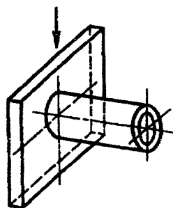
Рис.12. Нижнее положение при горизонтальном расположении оси трубы, привариваемой с поворотом
