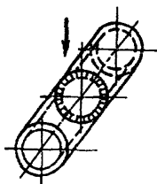
Рис.5. Нижнее положение при горизонтальном расположении оси труб, свариваемых с поворотом
