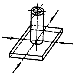
Рис.13. Нижнее положение при вертикальном расположении оси привариваемой трубы
