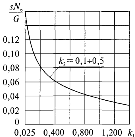
Рис. 7.8. Номограммы для вычисления усилий N_z , N_\phi в коллекторе при D_a/s = 9 \div 13 и a < b
