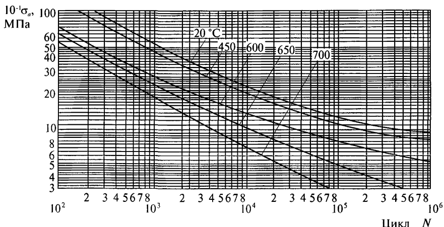
Рис. 5.4. Расчетные кривые малоциклового усталости аустенитных хромо- никелевых сталей
