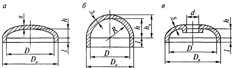
Рис. 3.2. Выпуклые днища:
