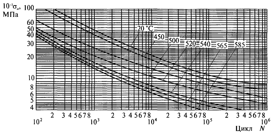
Рис. 5.3. Расчетные кривые малоциклового усталости низколегированных сталей марок 12X1MФ, 15X1M1Ф, 12MX и 15XM
