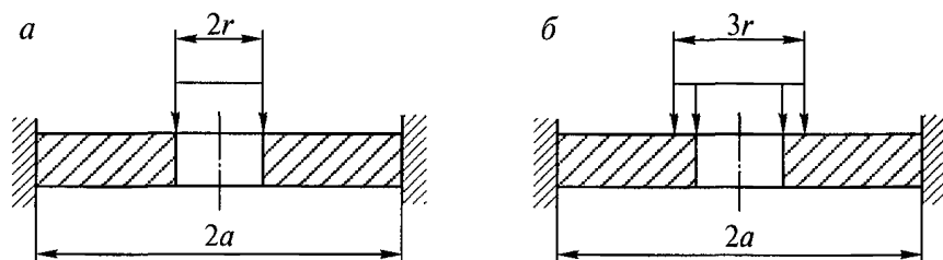
Рис. 10.8. Варианты нагружения:
