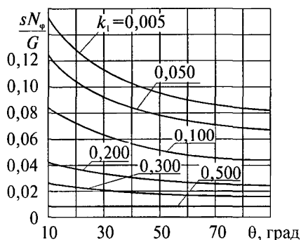
Рис. 7.6. Номограммы для вычисления усилий N_z , N_\phi в коллекторе при D_a/s = 14+35 и a > b
