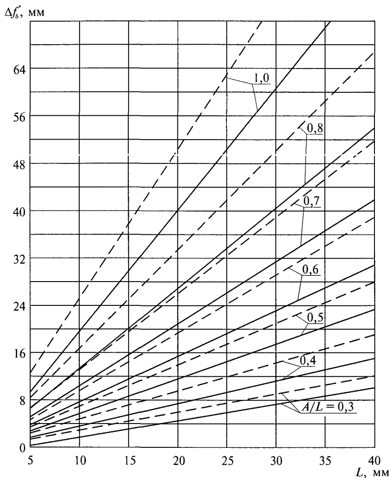
Рис. 10.6. Номограмма для определения максимальной разности прогибов пружин: — при нормальных условиях эксплуатации ( 1/500 ); - - - при сейсмическом воздействии ( 1/400 )
