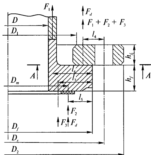
Рис. 8.4. Фланец с нажимным кольцом
