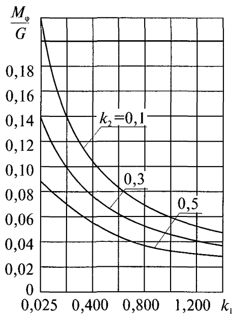
Рис. 7.9. Номограммы для вычисления моментов M_z , M_\phi в коллекторе при D_a/s = 9 \div 13 и a < b
