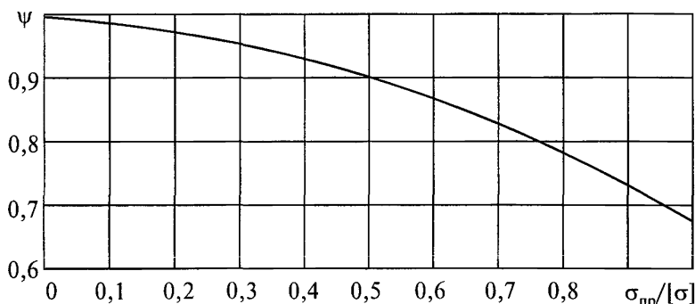
Рис. 5.11. Коэффициент \Psi
