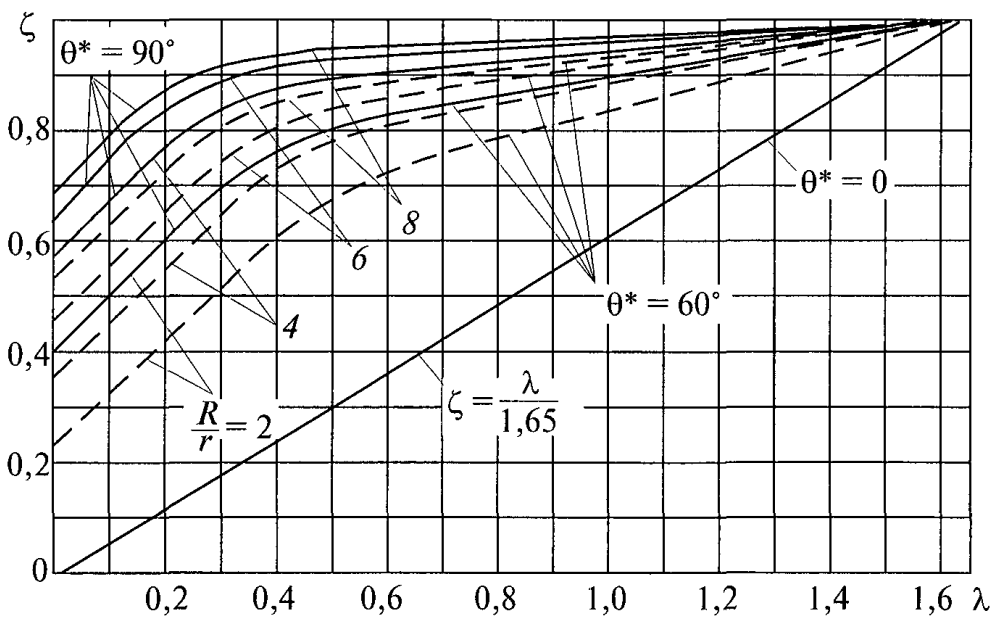
Рис. 5.8. Коэффициент \zeta
