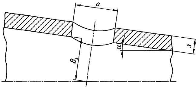
Рис. 4.11. Коническая деталь
