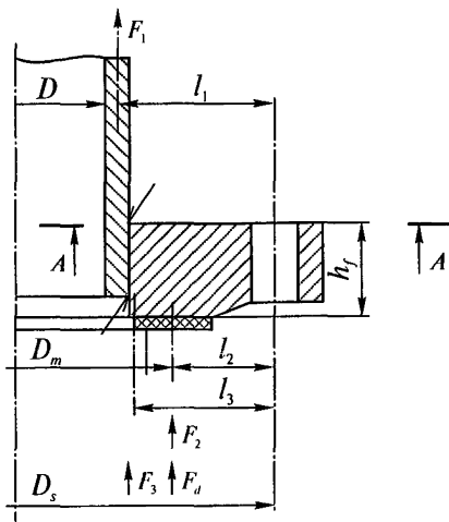
Рис. 8.6. Плоский фланец
