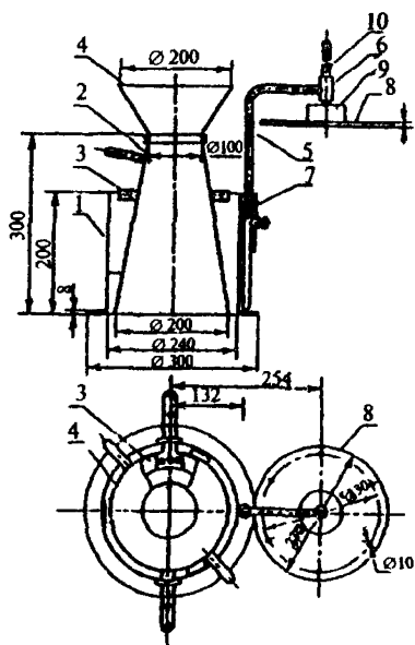
Рисунок 2 — Установка типа Вебе
