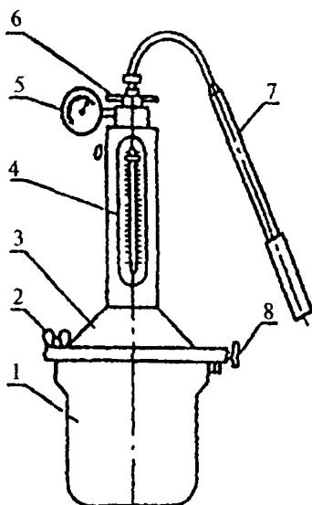
Рисунок 5 — Поромер
