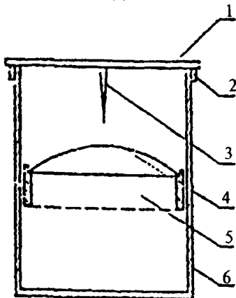
Рисунок 4 — Объёмомер
