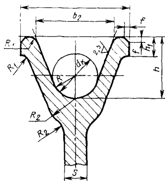
Профиль обода блока
