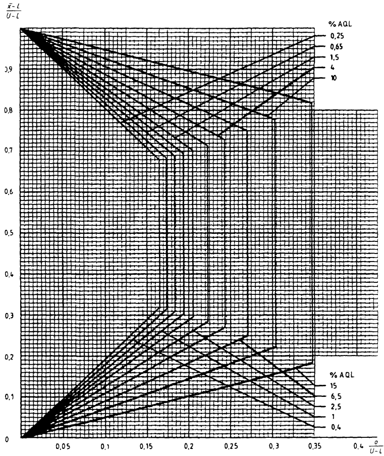
Диаграмма \sigma -Е — Кривые приемки для предельных значений с общим уровнем качества: \sigma -метод для кода объема выборки Е
