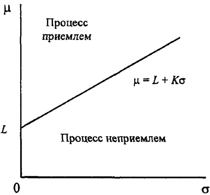
Рисунок 8 — Приемочная карта для нижнего предела поля допуска ( \sigma и \mu известны)
