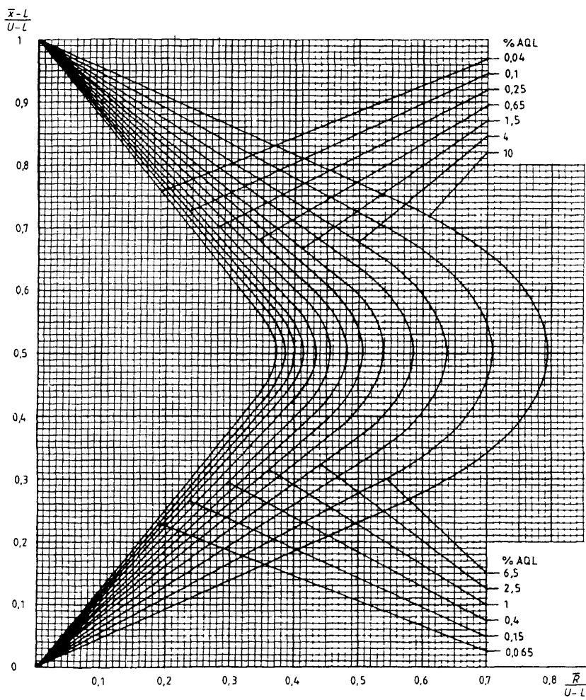
Диаграмма R-N — Кривые приемки для предельных значений с общим уровнем качества: R-метод для кода объема выборки N (объем выборки — 175)
