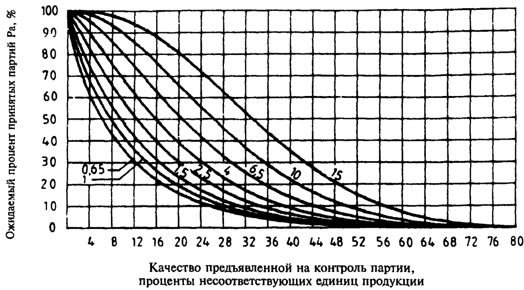
График VD — Оперативные характеристики для одноступенчатых выборочных планов контроля
