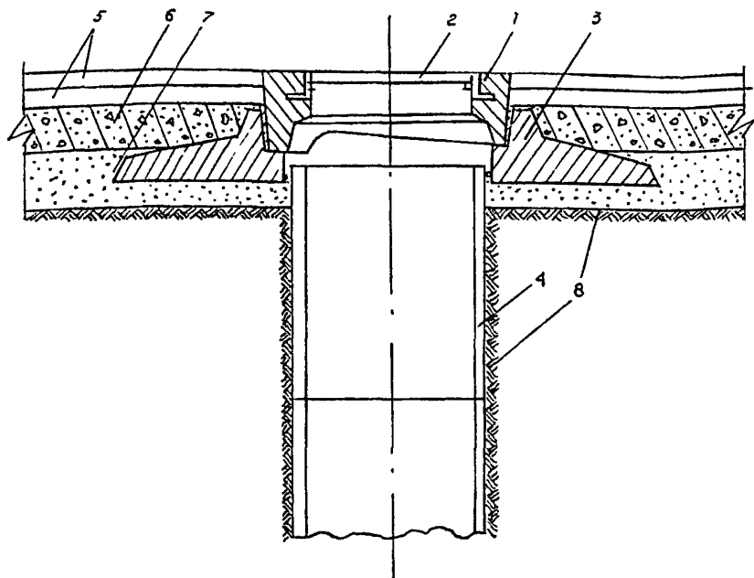
Рис. 2.3. Сопряжение оголовка колодца с дорожной одеждой и горловиной:
