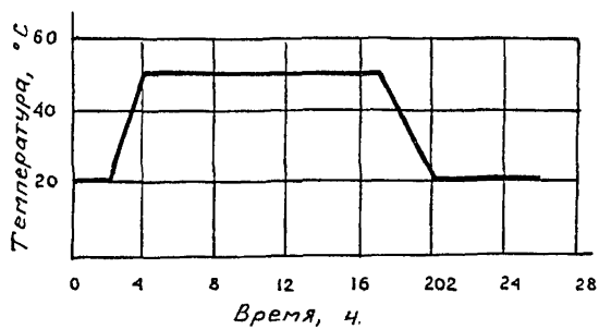
Рис. 3.1. Ориентировочный режим гидротермальной обработки железобетонных элементов сборного оголовка
