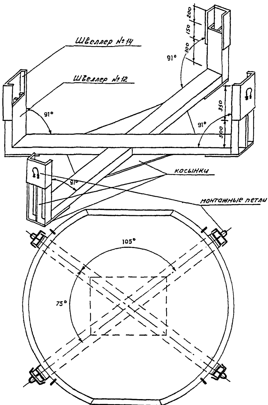
Рис. 4.1. Инвентарная оснастка для складирования и транспортировки оголовков
