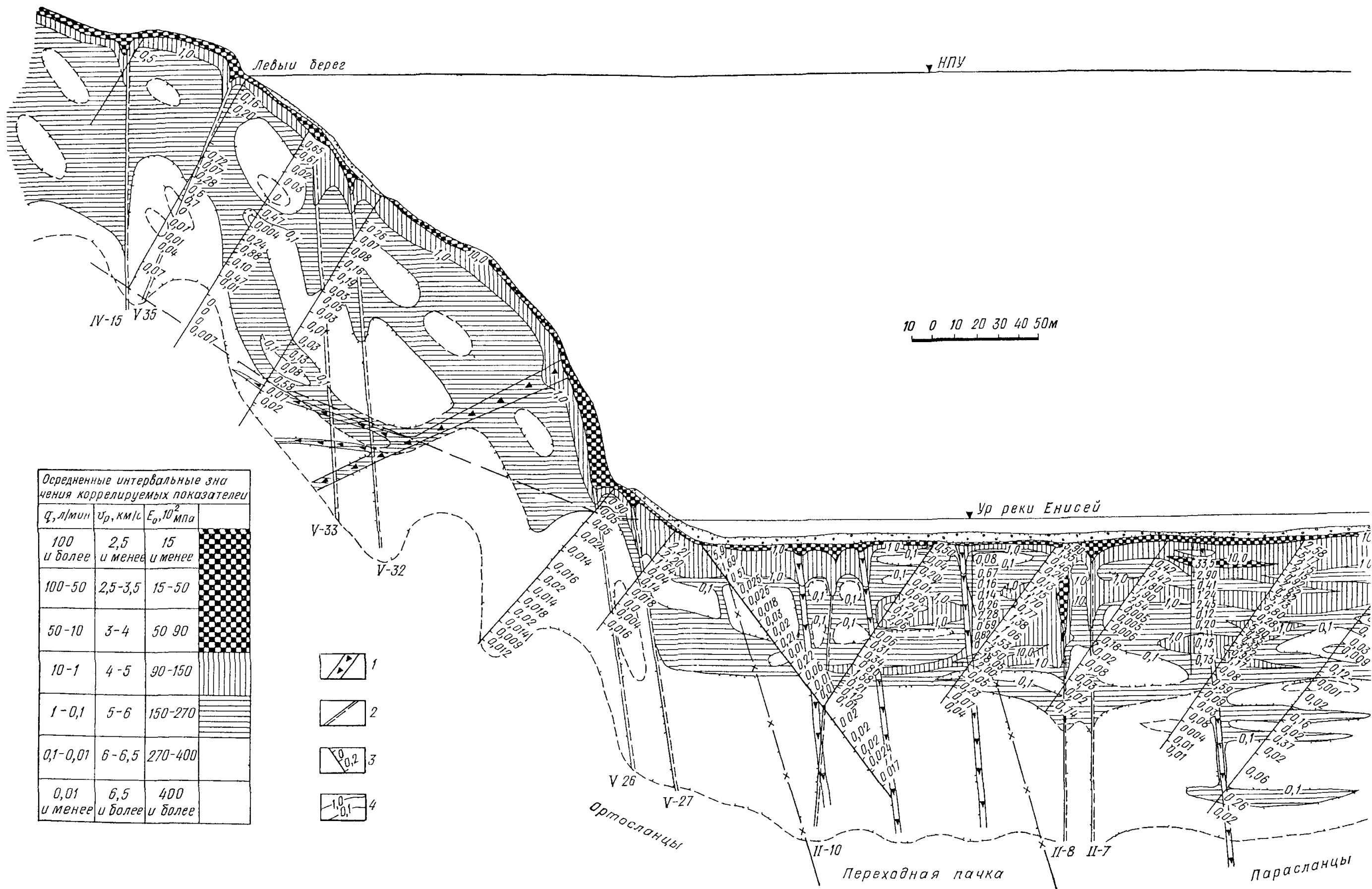
Рис. 3.9. Фрагмент уточненной модели водопроницаемости естественного скального массива. Разрез I—I по хорде арочно-гравитационной плотины Саяно-Шушенской ГЭС. 1 — дайки диоритов; 2 — тектонические нарушения и их номер; 3 — интервальные значения q (л/мин); 4 —
