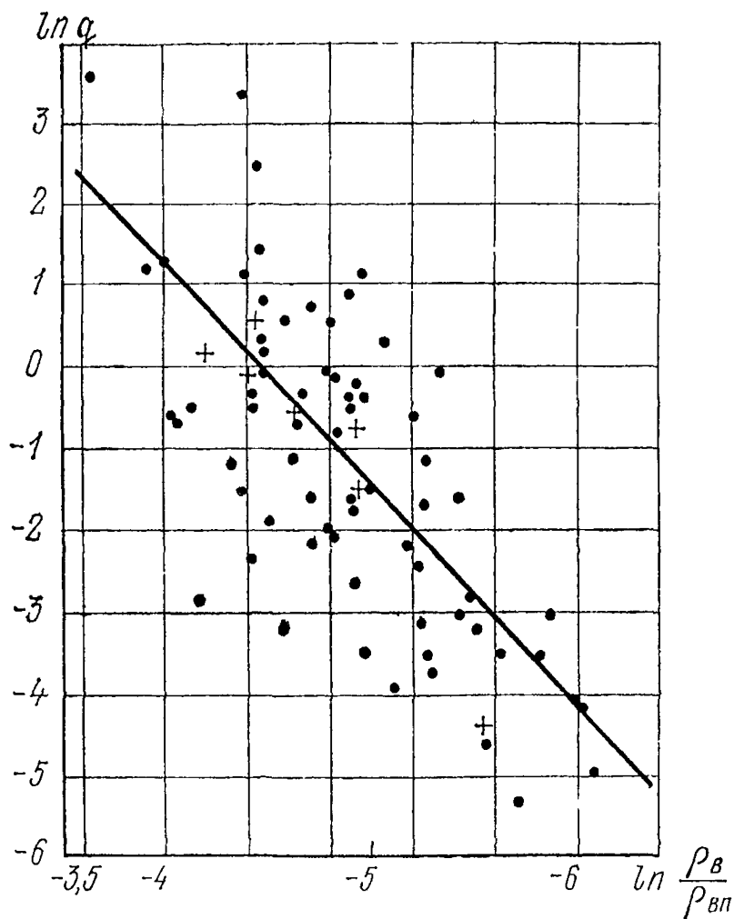
Рис 2.2 Связь q с обратной величиной относительного элект- рического сопротивления ( \rho_{vp}/\rho_v ) в массиве диоритов осно- вания Зейской ГЭС
