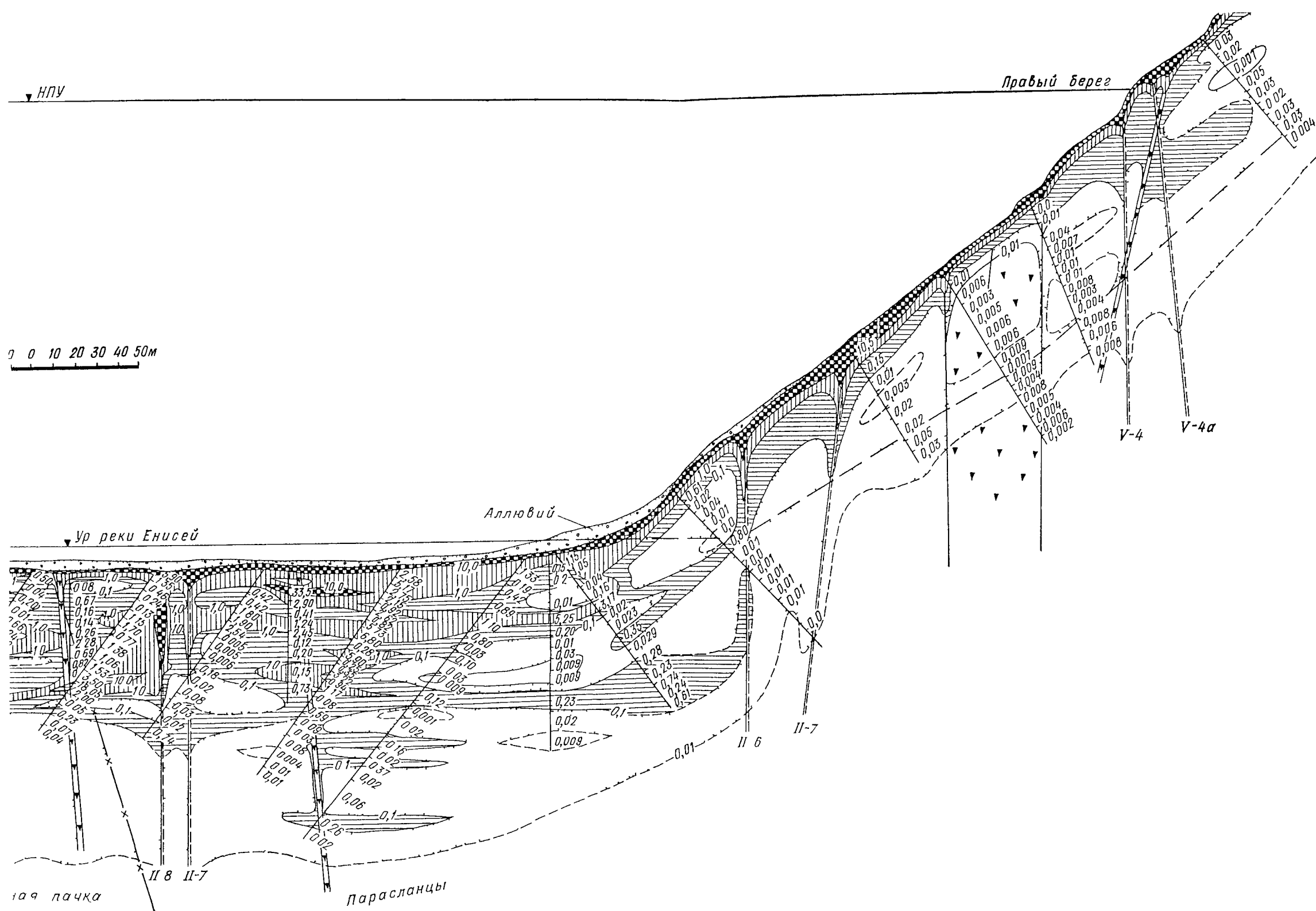
I по хорде арочно-гравитационной плотины Саяно-Шушенской ГЭС. Интерпретация с взаимовязкой данных опытно-фильтрационных и геофизических исследований.
