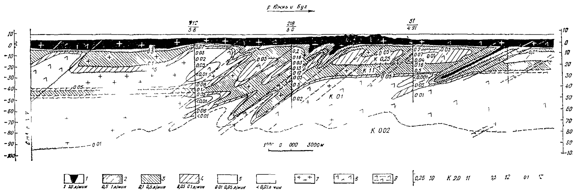
Рис 3.8 Водопроницаемость скального основания Константиновского гидроузла. Разрез по долине р Ю Буг 1 — q=1-10 л/мин, 2 — q=0,5-1 л/мин, 3 — q=0,1-0,5 л/мин, 4 — q=0,05-0,1 л/мин, 5 — q=0,01-0,05 л/мин, 6 — q<0,01 л/мин 7 — граниты, 8 — диориты, 9 — мигматиты, гнейсы, 10 — интервал опробования нагнетаниями и величины удельного водопоглощения, л/мин, 11 — расчетное значение коэффициента фильтрации м/сут, 12, 13 — границы зон с различными удельными водопоглощением и коэффициентом фильтрации (12 — установленные, 13 — предполагаемые)
