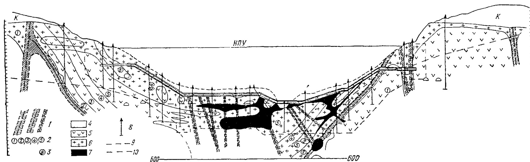
Рис 3-4 Схеа фильтрационной неоднородности пород основания плотины Чарвакской ГЭС
