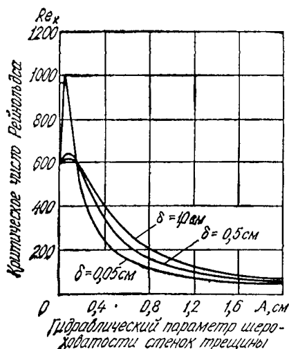
Рис 1-2 Графики изменения критического числа Рейнольдса потока воды в трещине в зависимости от гидравлического параметра шероховатости ее стенок (при t_{\text{в}} = 20^\circ\text{C} ) (по В. Н. Жиленкову)
