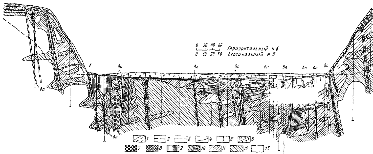
Рис 30 Фрагмент модели водопроницаемости скального основания Красноярской ГЭС
