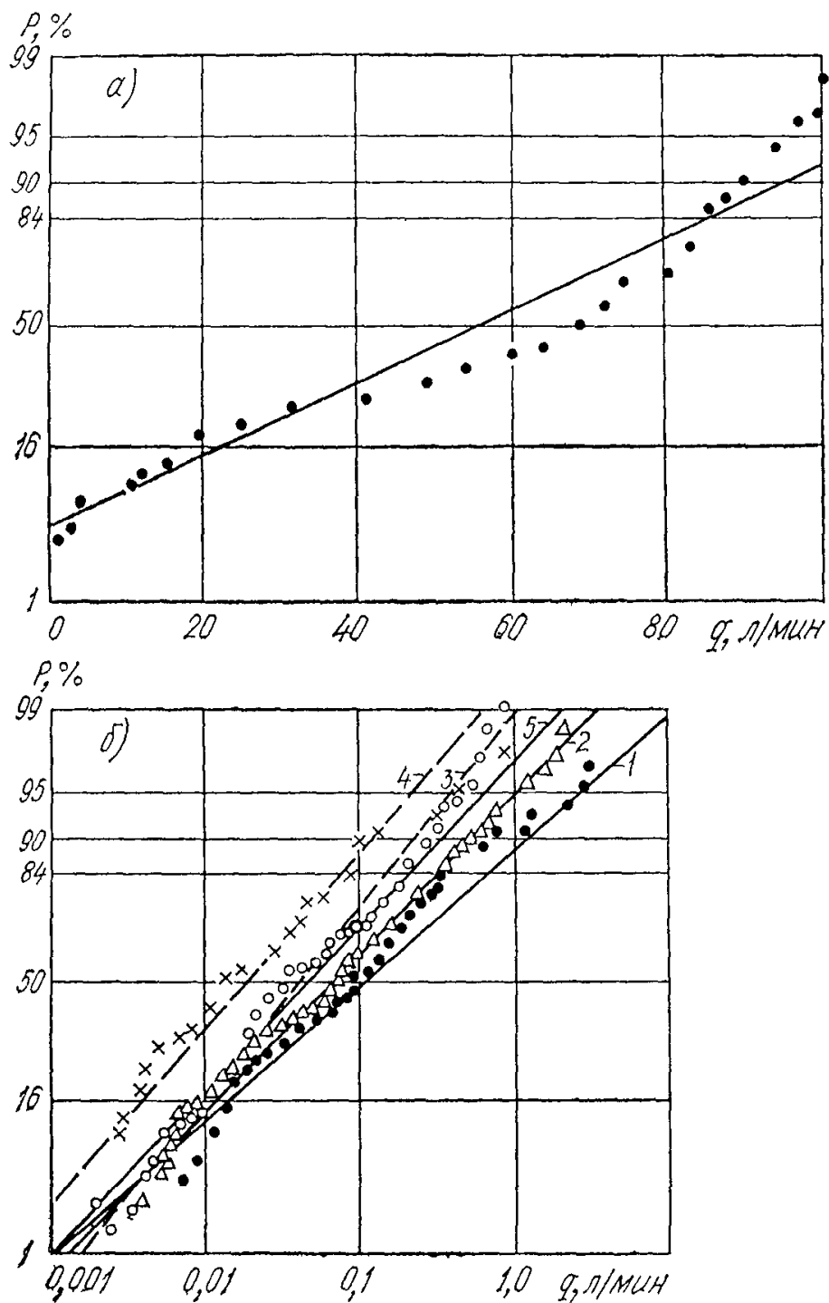
Рис. 17. Примеры распределения значений q на вероятностной (а) и логарифмически-вероятностной (б) бумаге: а — известняки основания Ингурской ГЭС (зоны тектонических нарушений), выборка № 21; б — парасланцы вне зон тектонических нарушений — основание Саяно-Шушенской ГЭС, выборка № 1 1 — интервал глубин H = 0 \div 15 м; 2 — H = 15 \div 35 м; 3 — H = 35 \div 75 м; 4 — H = 75 \div 100 м; 5 — H = 0 \div 100 м (в целом); [17].
