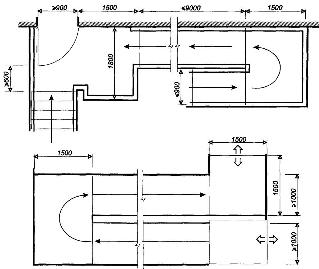
Промежуточные площадки
