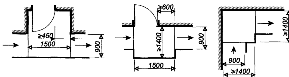
Конечные площадки
