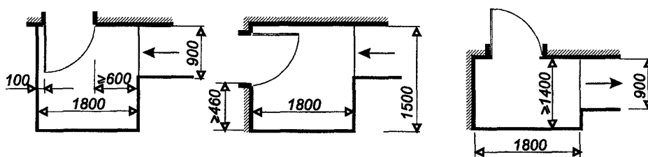
Конечные площадки
