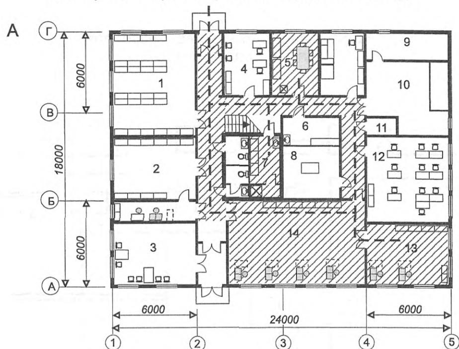
Мастерская по ремонту бытовой радиоаппаратуры
