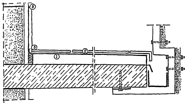
Рис. 4.9. Балконы и террасы. Гидроизоляция и ремонт: 1-Аквафин-2К; 2-Унифлекс -2К; 3-Ескосил
