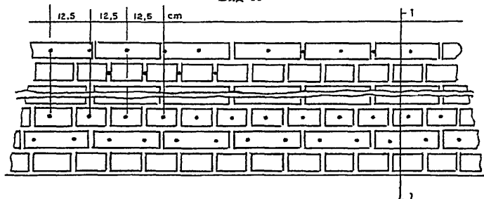
Разрез 2-2 1-1
