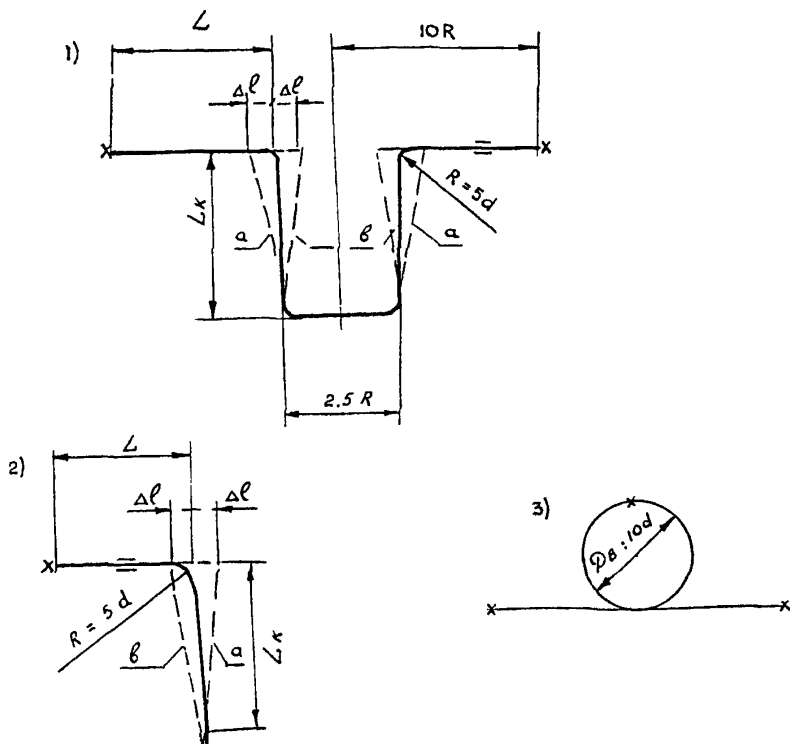
Рис. 7. Устройство компенсаторов
