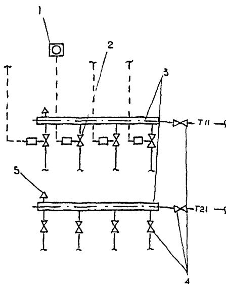
Рис. 3. Распределительный коллектор систем отопления:
