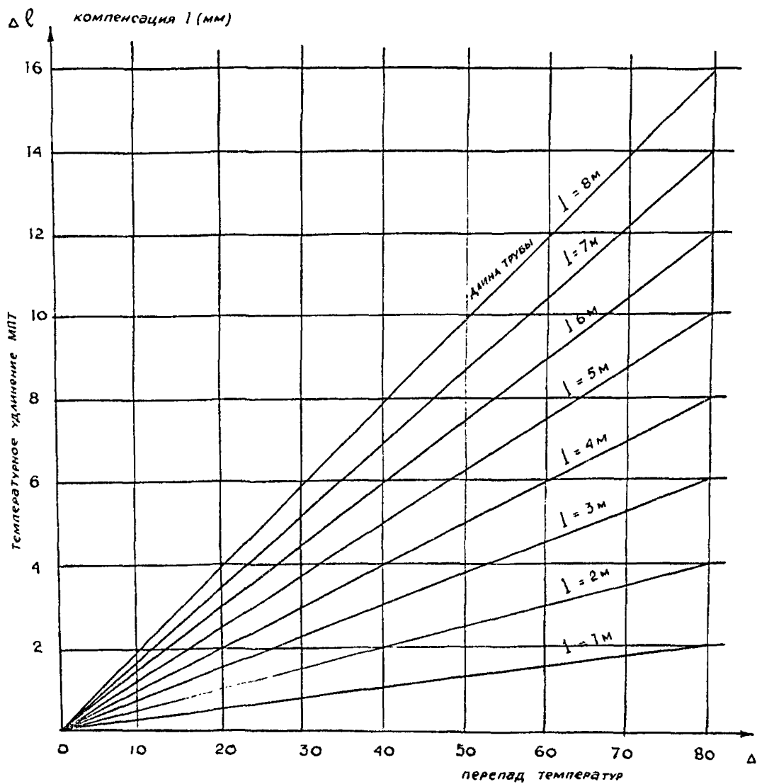
Рис. 6. Диаграмма уплотнения МПТ
