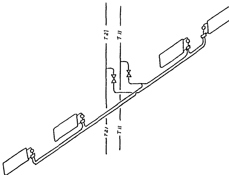
Рис. 2. Система отопления с горизонтальными однетрубными ветками для группы последовательно соединенных отопительных приборов
