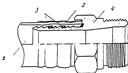
Рис. 11в. Соединение с обжимной втулкой:
