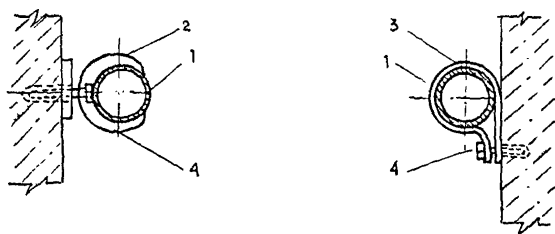
Рис. 12. Крепление труб к стенам и перегородкам:
