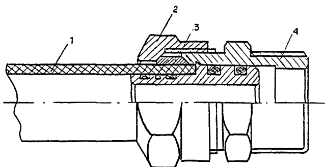
Рис. 11б. Соединение с накладной гайкой и разрезным кольцом:
