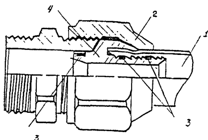
Рис. 11а. Соединение с накладной обжимной гайкой:
