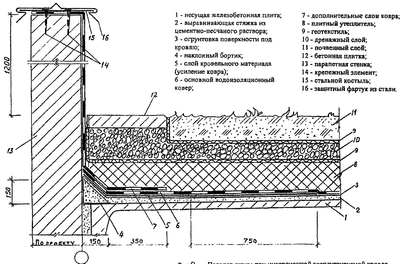
Рис.9 Парапет стены при инверсионной эксплуатируемой кровле.
