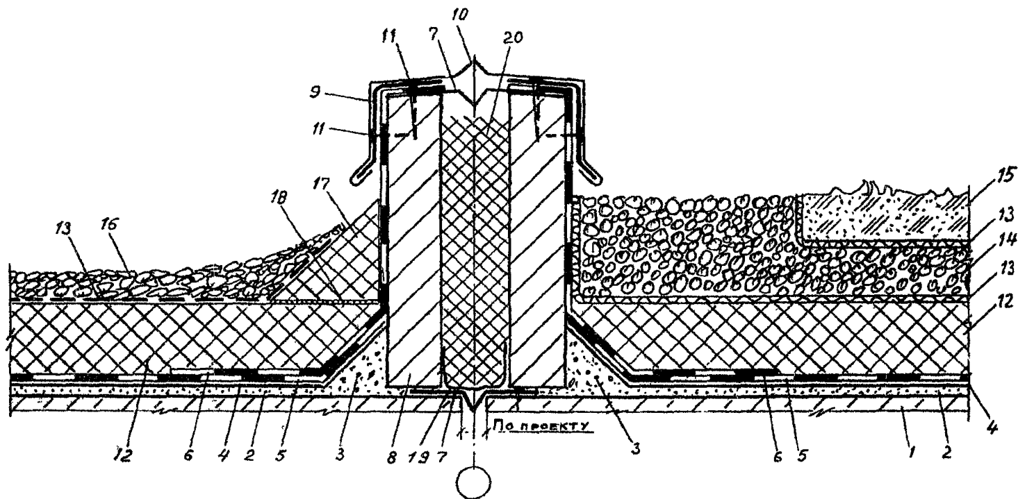
Рис.6 Деформационный шов при инверсионной эксплуатируемой кровле.
