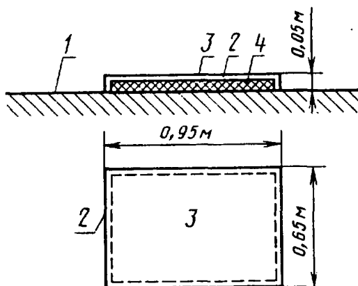
1 — стена; 2 — деревянная рама; 3 — фанера; 4 — стекловата или минераловата
