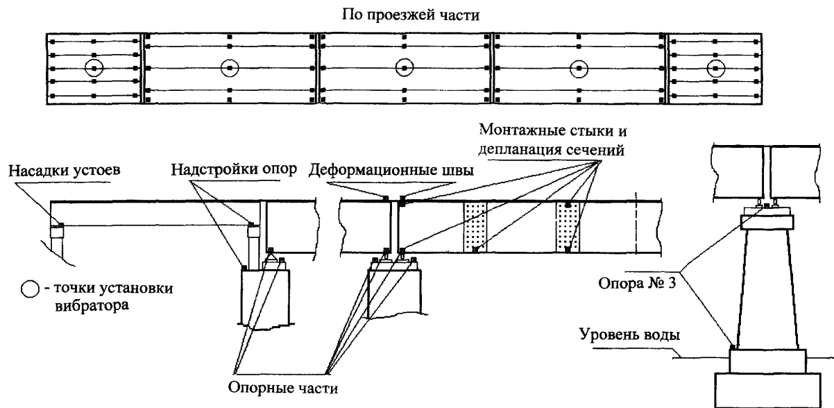
Схема нагружения и измерений при вибродиагностике большого моста
