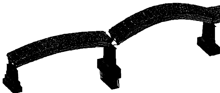
Форма колебаний МКЭ-модели на частоте 2.2 Гц
