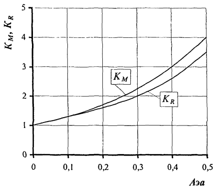
Рис. Д.3 – Графики зависимости коэффициентов K_M и K_R от эффективного коэффициента сейсмичности A_{\text{э}a} .
