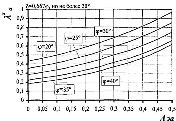
Рис.Д.1 – График зависимости коэффициента горизонтальной составляющей активного остаточного давления \lambda^s_a от эффективного коэффициента сейсмичности A_{эа}
