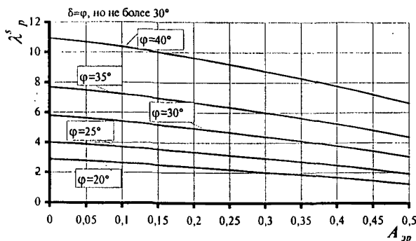
Рис.Д.2 – График зависимости коэффициента горизонтальной составляющей пассивного остаточного давления \lambda^s_p от эффективного коэффициента сейсмичности A_{эп}
