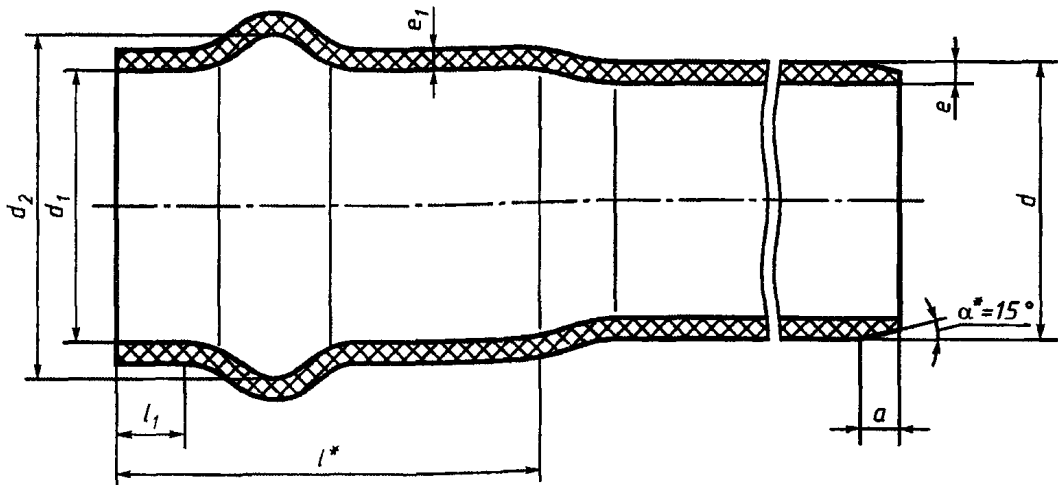
* Размеры являются справочными. a — длина фаски; d — номинальный наружный диаметр трубы; d_1 — внутренний диаметр раструба; d_2 — внутренний диаметр раструба в зоне установки уплотнительного кольца; e — номинальная толщина стенки трубы; e_1 — толщина стенки раструба; l — длина раструба; l_1 — длина раструба до канавки под уплотнительное кольцо; \alpha — угол фаски
