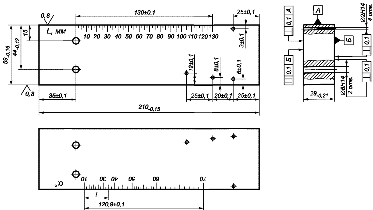
Рисунок 3 — Стандартный образец СО-2Р
