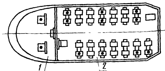
1—кабина экипажа; 2—салон Черт. 5
