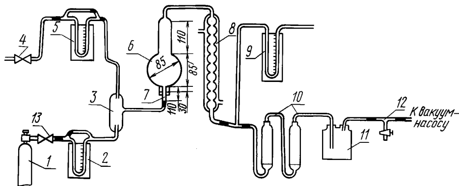
Прибор для определения массовой доли общей серы
