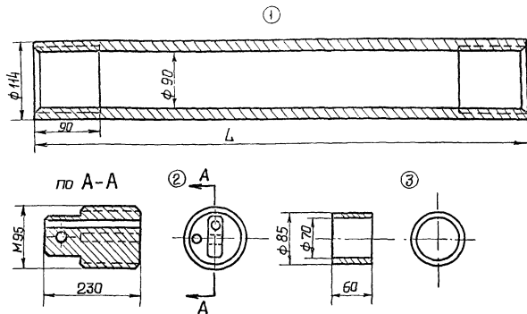
Рис. 1 Конструкция углеграфитового анода
