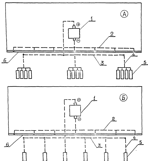
Рис. 2 Схемы анодных линий
