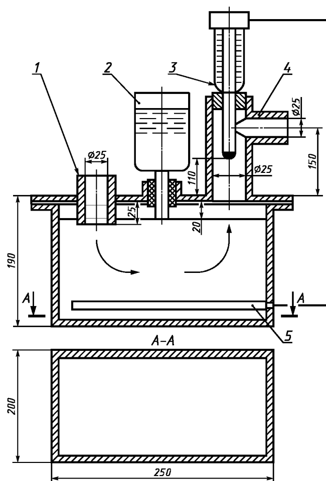
1 — штуцер, направленный к ИЛ; 2 — пополняющий резервуар; 3 — терморегулирующее устройство; 4 — штуцер, направленный к тройнику; 5 — электронагреватель
