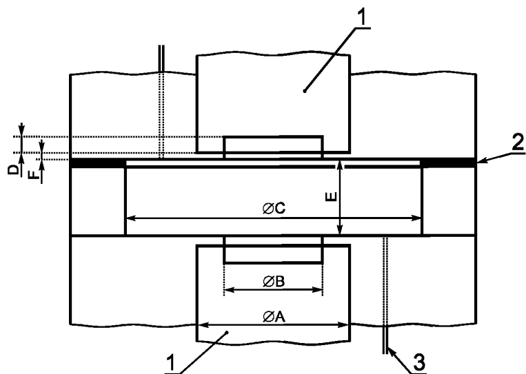
1 — микрофон; 2 — изолятор; 3 — капиллярные трубки
