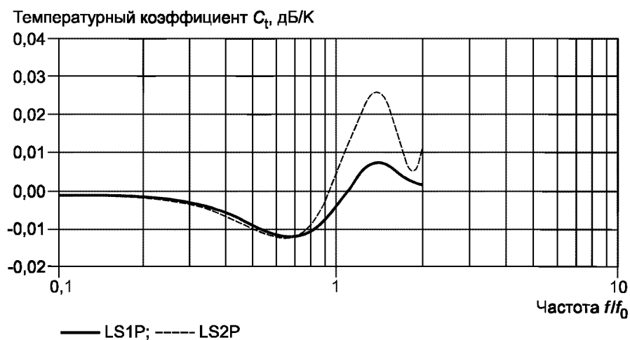
Рисунок В.2 — Типичная форма зависимости составляющей C_t температурного коэффициента чувствительности по свободному полю от безразмерной частоты f/f_0 ( f_0 — резонансная частота микрофона), вызванной изменениями импеданса воздуха в замкнутых полостях и около микрофона, для микрофонов типов LS1P и LS2P
