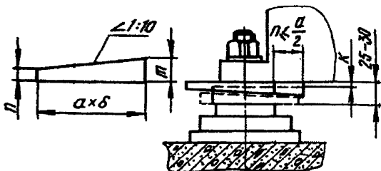
Рис.7. Клиновые подкладки
