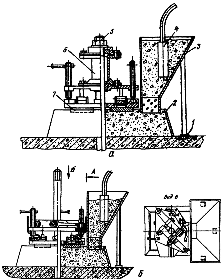
Устройство для установки опорных элементов на фундаменте:
