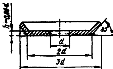
Рис.1. Установочная шайба (наружный диаметр развертки лабы 3,4d ; материал - Ст3)
