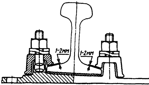
Рис. 2.5. Рельсовое скрепление КБ с подрезанными лапками клемм (с опиранием клемм на ребры рельсовых подкладок)
