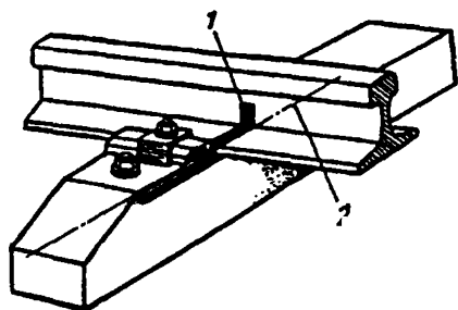
Рис. 4.1. "Маячная" шпала для контроля угона пути:
