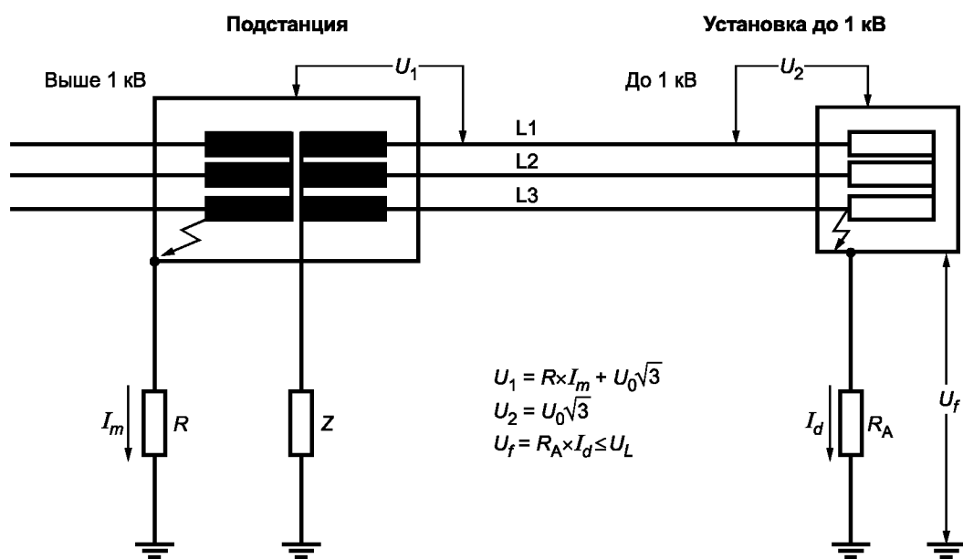
Рисунок 44F — IT-системы, пример с1)
