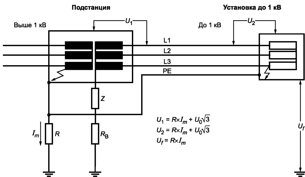
Рисунок 44J — IT-системы, пример е1)
