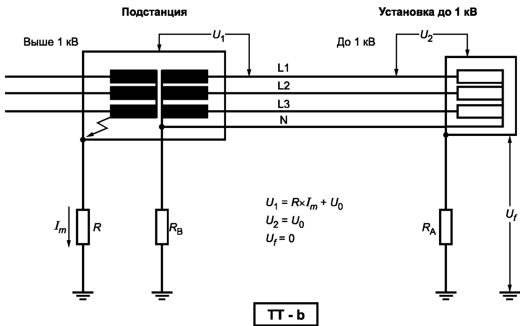
Рисунок 44С — ТТ-системы
