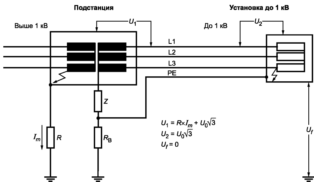
Рисунок 44Н — IT-системы, пример d)
