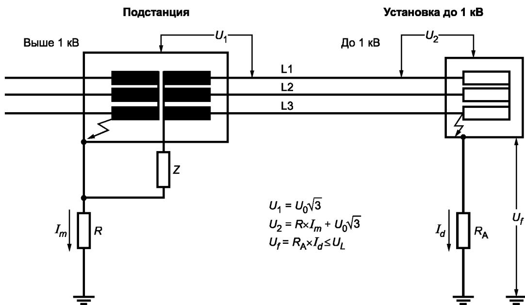
Рисунок 44Е — ИТ-системы, пример б)
