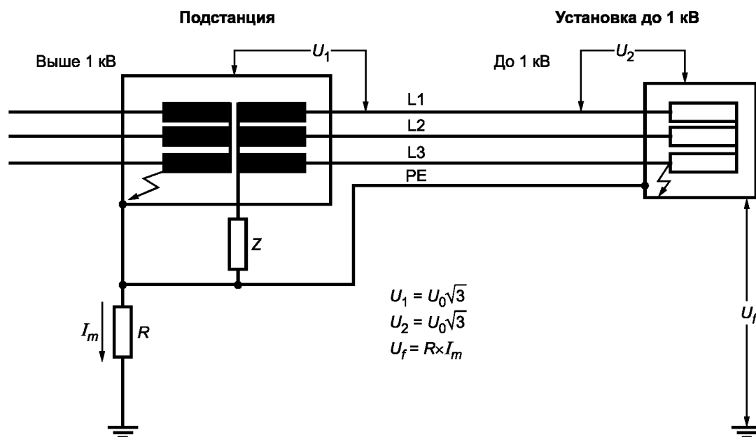
Рисунок 44D — IT-системы, пример а)
